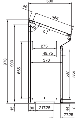
Przekrój A - A
