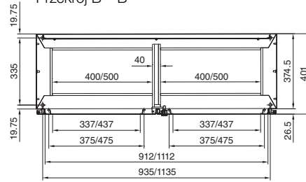
Przekrój B - B
