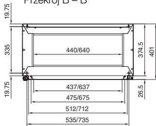
Przekrój B - B
