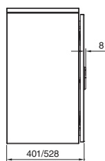
1-delat utförande
