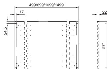
Montageplåt
