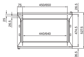
Montageplåt
