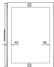
Montagehålbild
