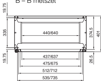
B – B metszet
