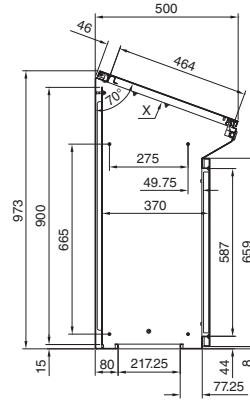
A – A metszet
