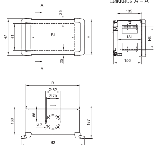
Leikkaus A – A
