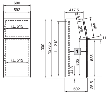
带较高的前门 TP2695.500
