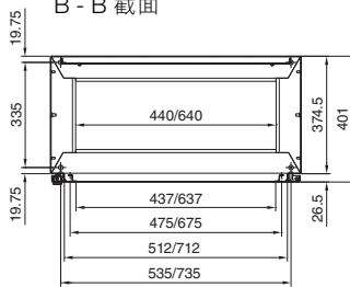
B - B 截面
