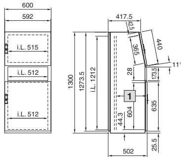
带较矮低的前门 TP2694.500
