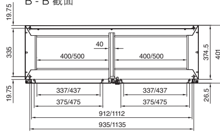
B - B 截面
