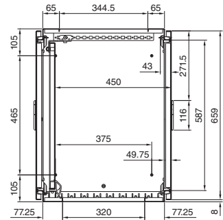
A - A 截面
