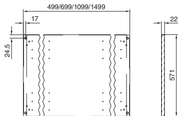
安装板
