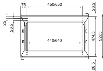
安装板
