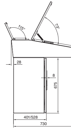
2 段式结构
