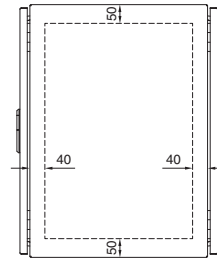
安装开口截面
