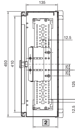
A - A 截面
