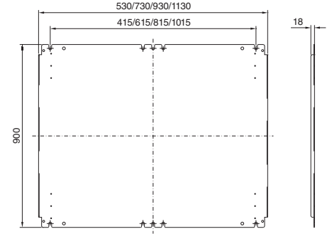
Montaj plakası
