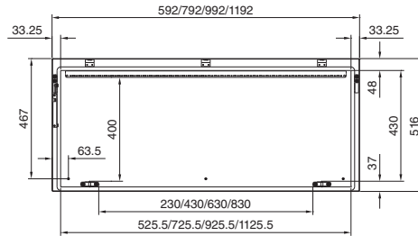
X yönünde görünüm
