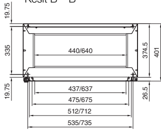
Kesit B - B
