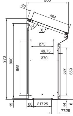
Kesit A - A
