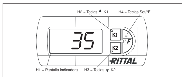
Figura 6.1 Regulación electrónica
