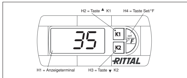
Abb. 6.1 Elektronische Regelung
