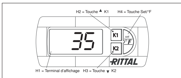
Fig. 6.1 Régulation électronique
