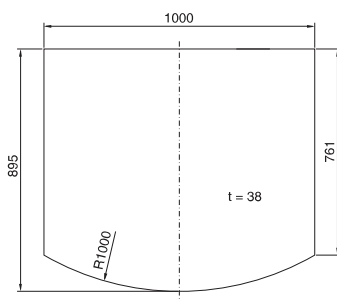
Arbeitsplatte IW 6902.100
