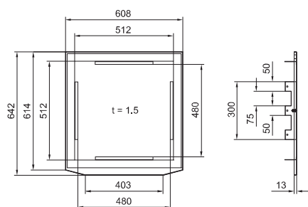
Dach IW 6902.400
