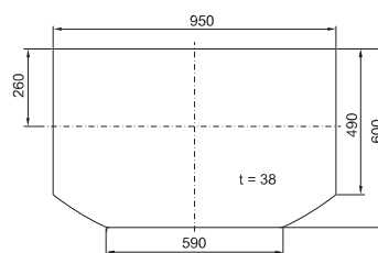
Arbeitsplatte, vorbereitet für Standfuß IW 6902.310
