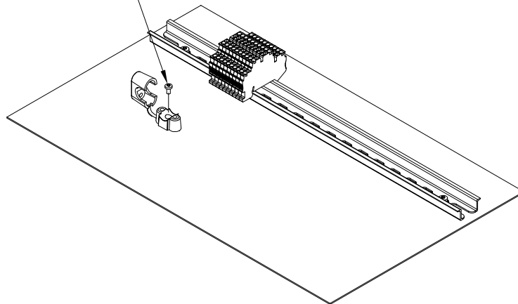
Befestigungsschraube M4x8 Fixing screw M4x8
