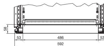
Particolare Y
