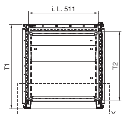
Sezione B – B
