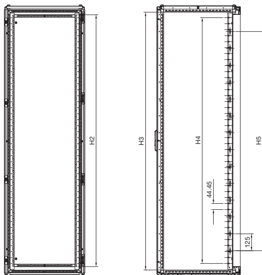
Vue de face sans cadre avant
