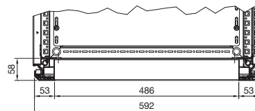
Détail Y
