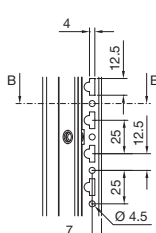
Sektion B - B
