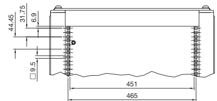
Detalj Y
