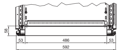
Detalj Y
