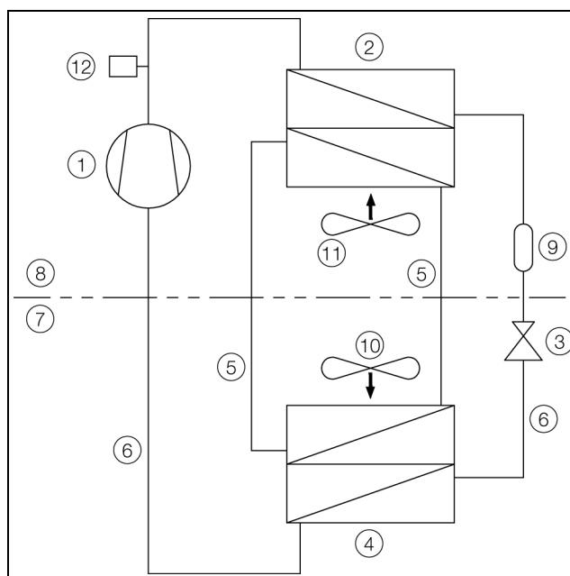
Fig. 1 : circuit frigorifique
