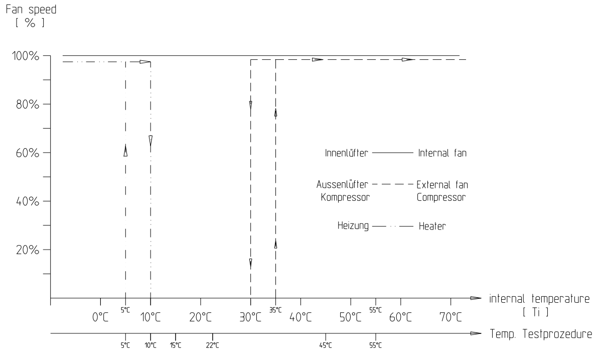
Abb. 4.1 Funktionsdiagramm
