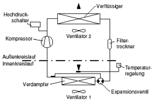
Abb. 8.1 Funktionsprinzip
