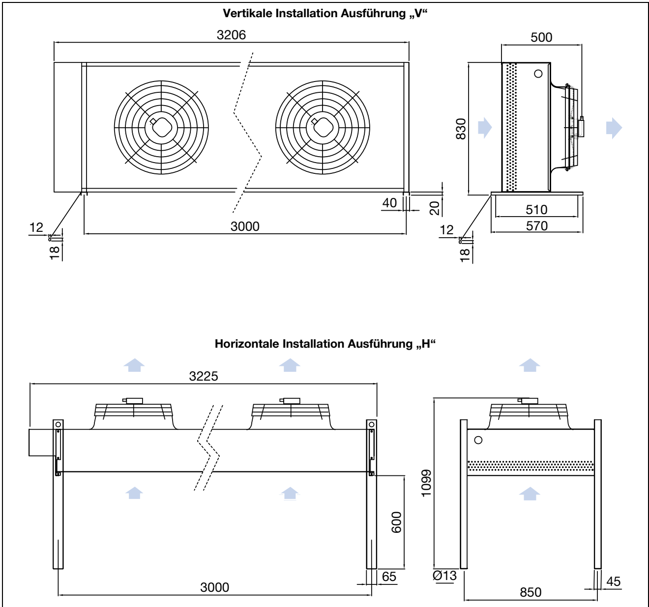
Abb. 74: Aufstellplan des Hochtemperatur-Verflüssigers (3311.XXX)
