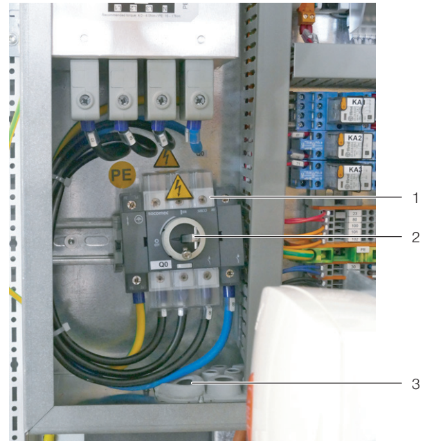
Abb. 28: Geöffnete Elektronikbox
