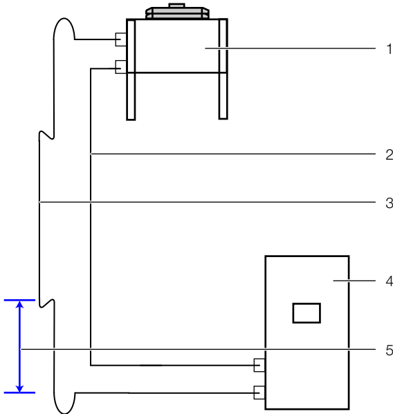
Abb. 21: Ölhebboegen
