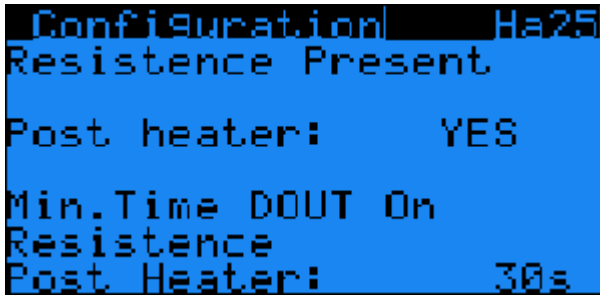
Abb. 56: Menü „Ha25“
