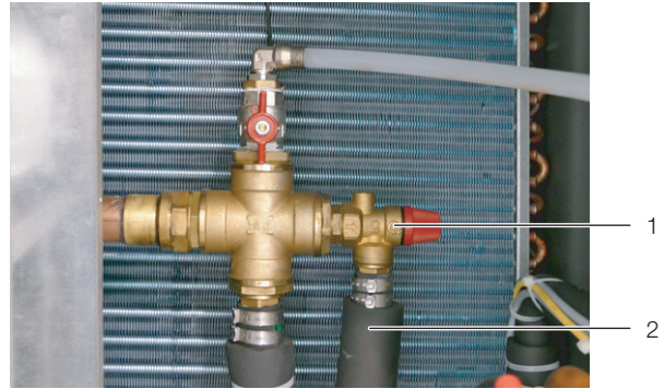
Abb. 27: Sicherheitsventil auf der Rückseite
