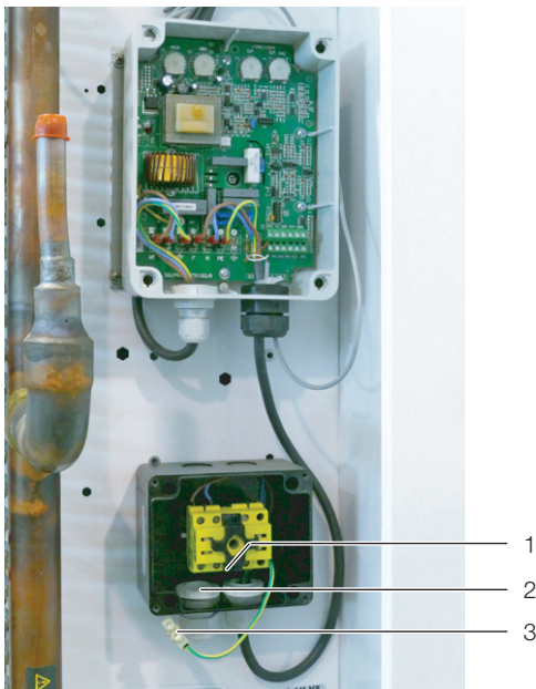
Abb. 30: Elektroanschluss am externen Verflüssiger
