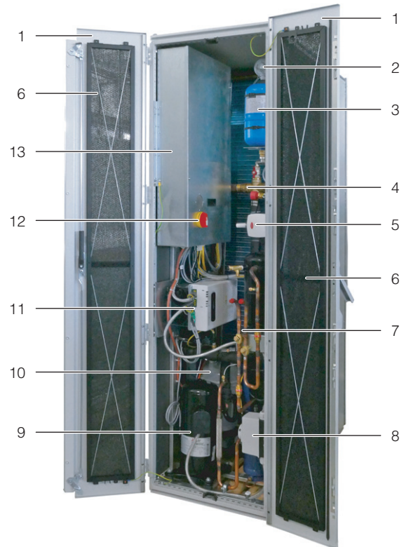
Abb. 4: LCP DX/FC Rückseite – Rücktüren geöffnet
