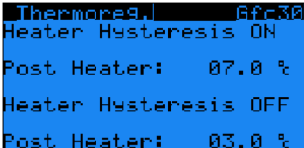
Abb. 57: Menü „Gfc30“
