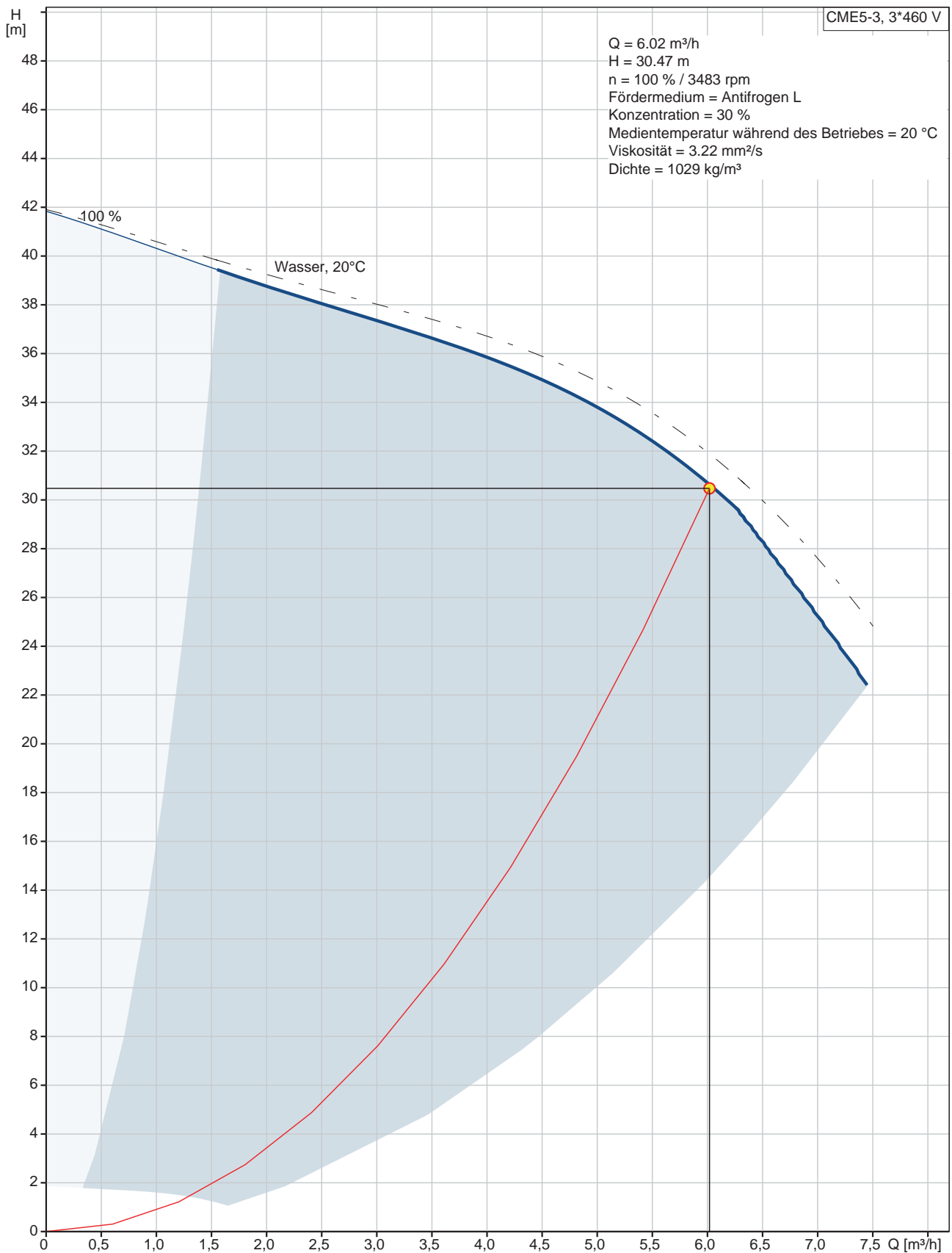
Abb. 81: Kennlinie Kühlwasserpumpe
