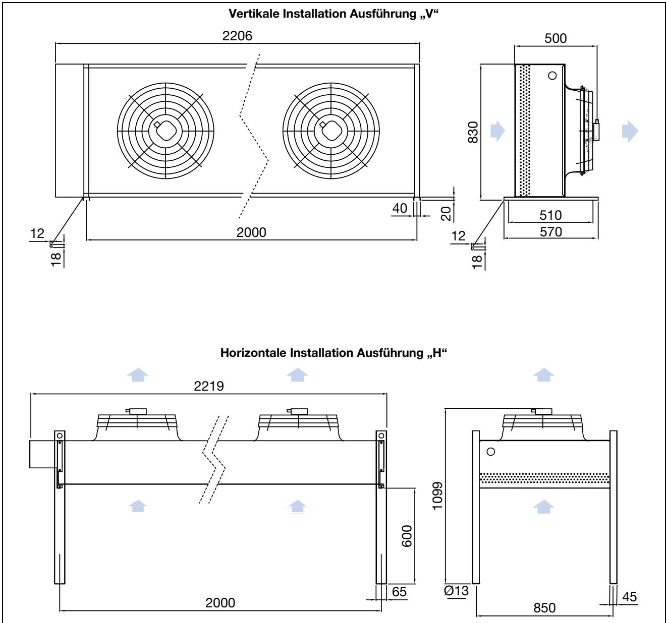
Abb. 72: Aufstellplan des Standard-Verflüssigers 3311.370
