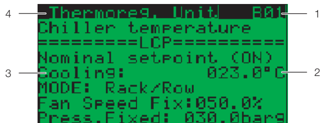
Abb. 38: Menü „Setpoint“
