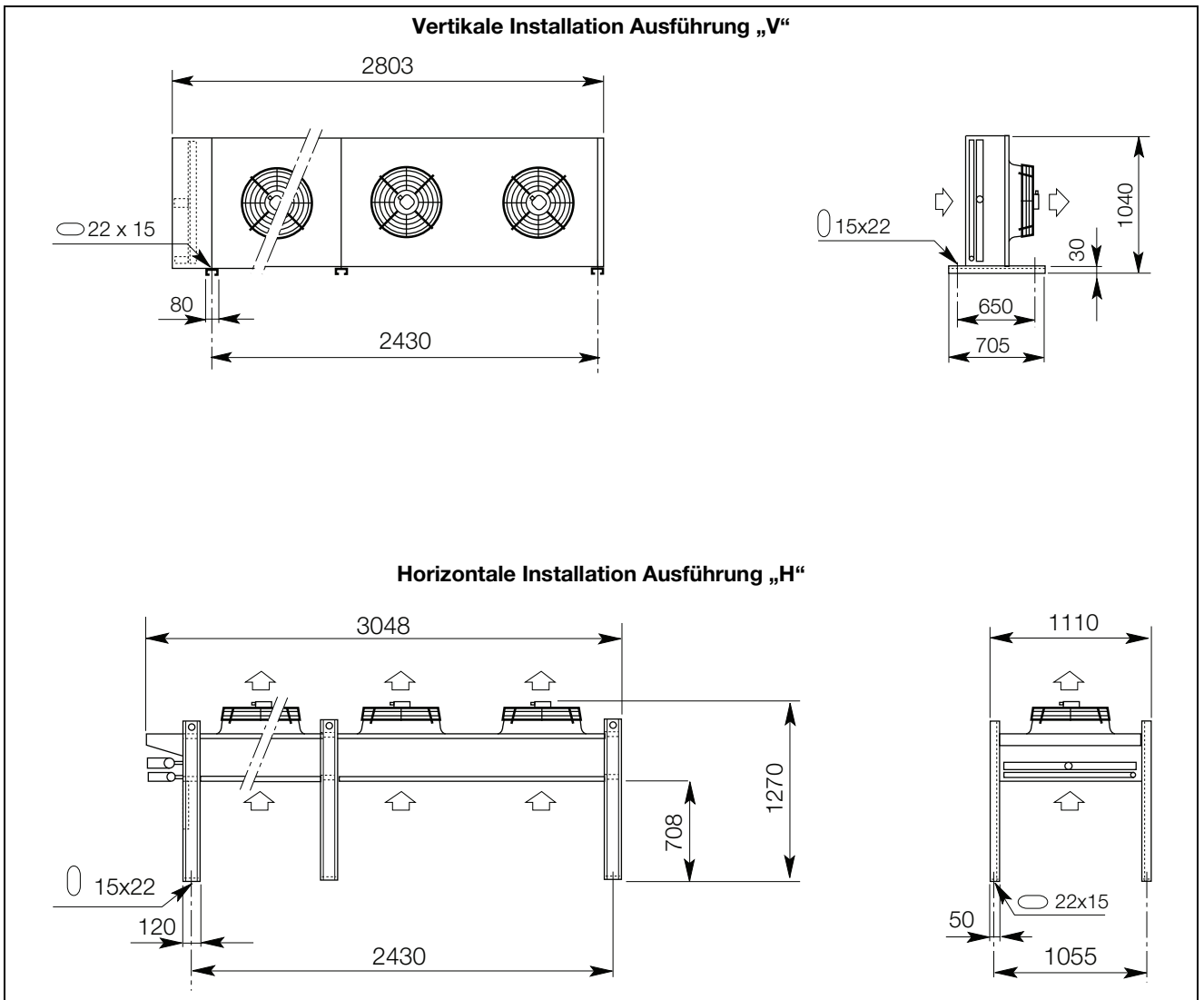
Abb. 73: Aufstellplan des Verflüssigers zur indirekten Freikühlung (3311.380)
