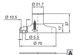
A Joint d'étanchéité
