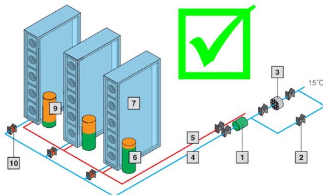
Рис. 50: Распределение холода с гидравлической балансировкой
