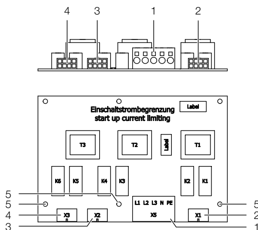
Рис. 94: Ограничитель пускового тока – задняя сторона/вид спереди
