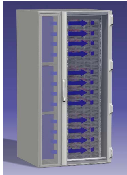
Рис. 5: LCP Rack с одним серверным шкафом
