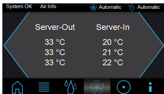
Рис. 65: Страница "Air-Info"
