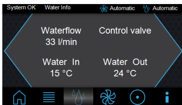
Рис. 64: Страница "Water-Info"
