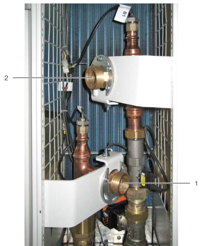
Рис. 46: Подключение холодной воды
