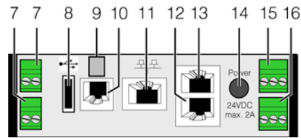
Рис. 58: Блок управления Liquid Cooling Package (CMC III PU) – задняя сторона
