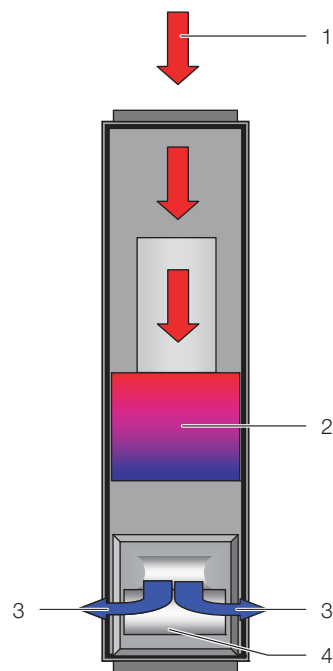
Рис. 2: Ток воздуха в LCP Inline – вид сверху
