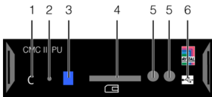
Рис. 57: Блок управления Liquid Cooling Package (CMC III PU) – передняя сторона
