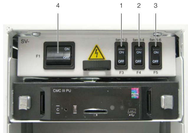
Рис. 13: Блок предохранителей с главным выключателем
