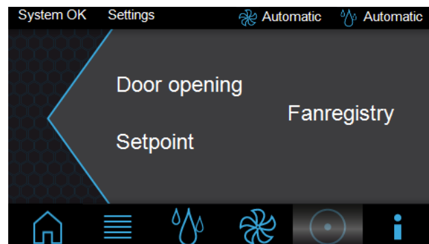
Рис. 66: Страница "Settings"
