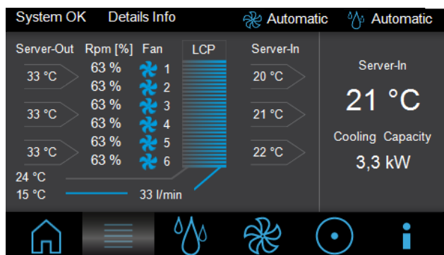
Рис. 63: Страница "Details"
