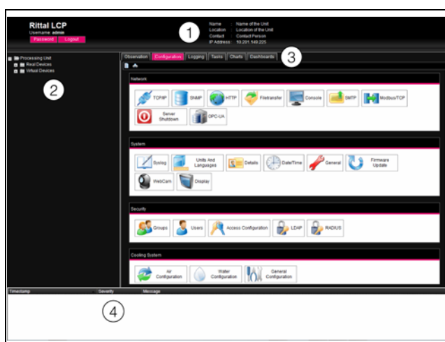
Рис. 74: Структура страницы
