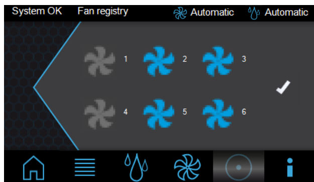
Рис. 71: Страница "Fanregistry"
