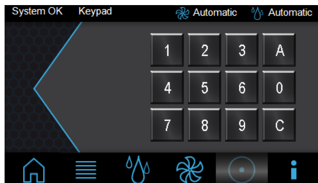
Рис. 70: Страница "Keypad"
