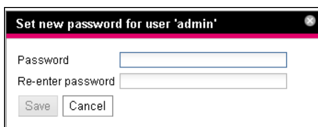
Рис. 82: Изменение пароля
