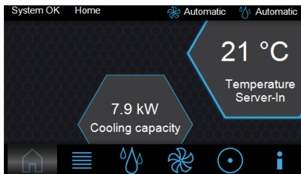
Рис. 60: Страница "Home"
