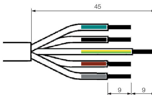
Рис. 40: Размеры снимаемой изоляции кабеля и отдельных проводов
