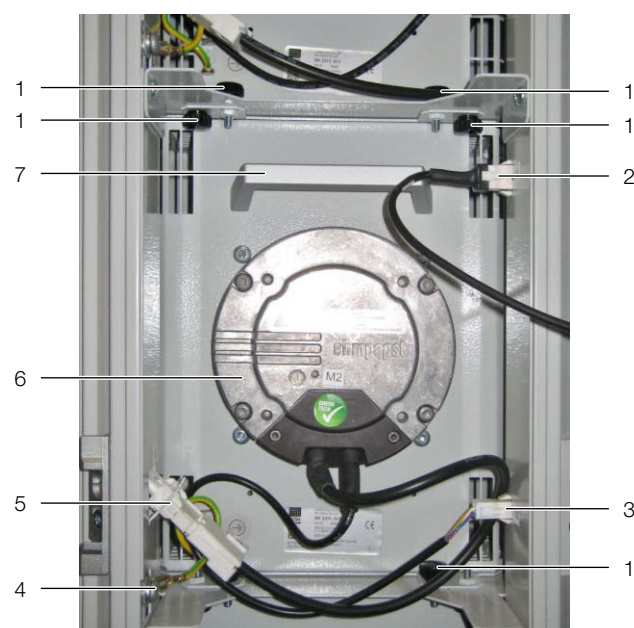
Рис. 15: Вентиляторный модуль в модульном отсеке – исполнение у LCP Inline и LCP Rack
