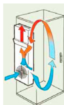
Applicazione con scambiatore di calore aria/aria
