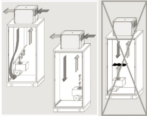
Evacuazione acqua di condensa in assenza di resistenza anticondensa
