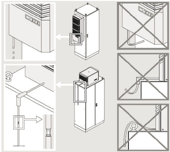
Evacuazione acqua di condensa in assenza di resistenza anticondensa
