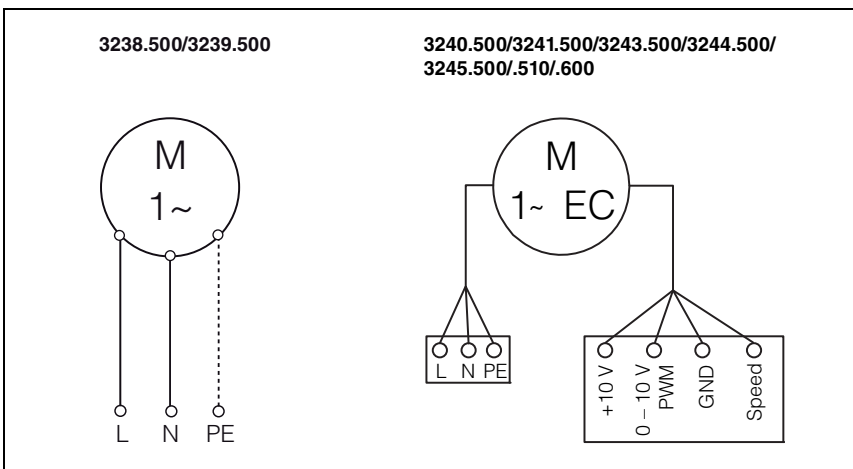
Рис. 11: Схемы подключения
