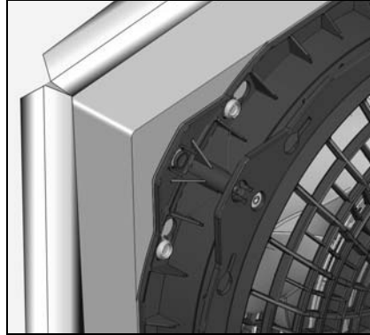
Рис. 10: ЭМС-контактные пленки
