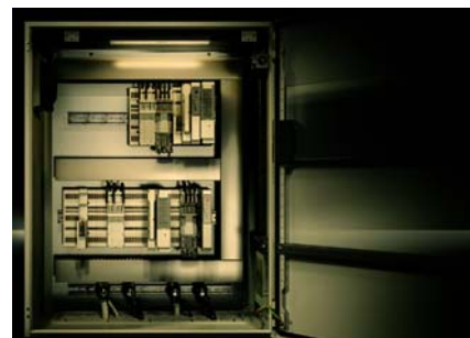
RiLine Compact består av en basplatta i vilken beröringsskyddade samlingskenor är monterade.
