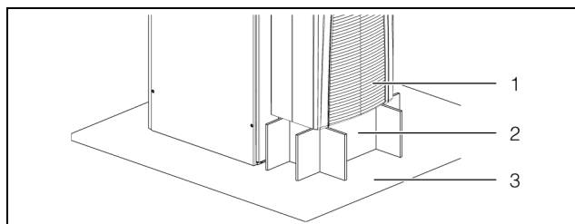
Afb. 4: Transportbeveiligingen
