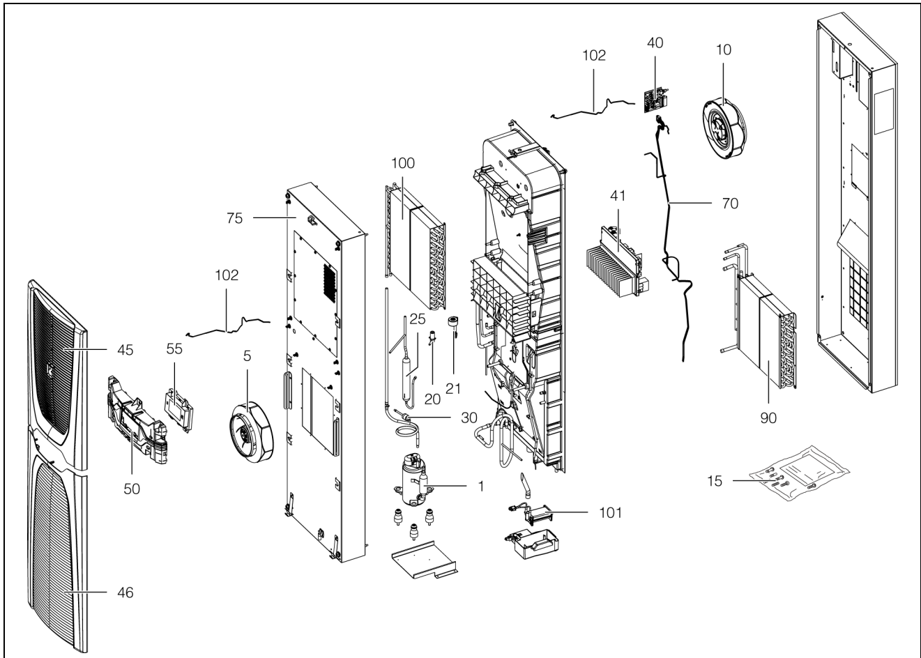
Afb. 37: Reservedelen (voorbeeldweergave)
