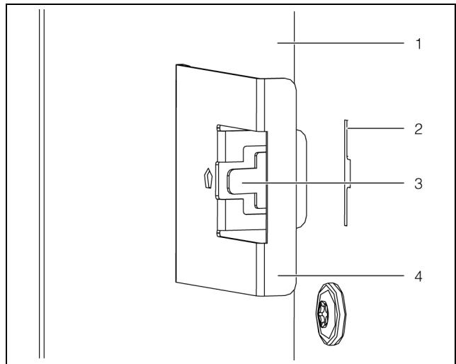
Afb. 35: Losmaken van de veerklemmen
