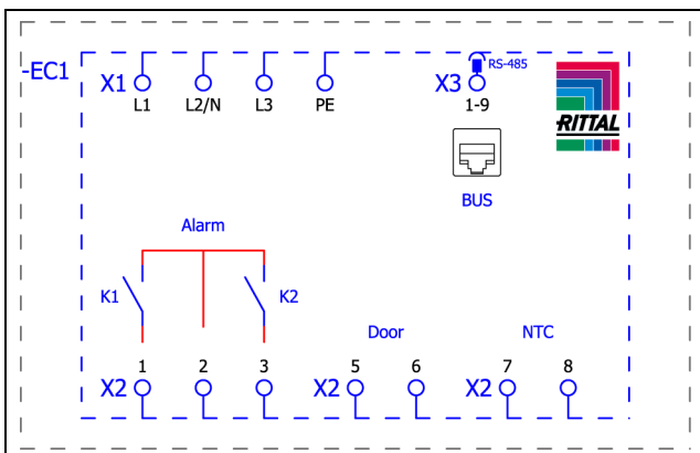
Afb. 17: Schakelschema SK 3184837, SK 3185x3x, SK 3186x3x en SK 3187x3x
