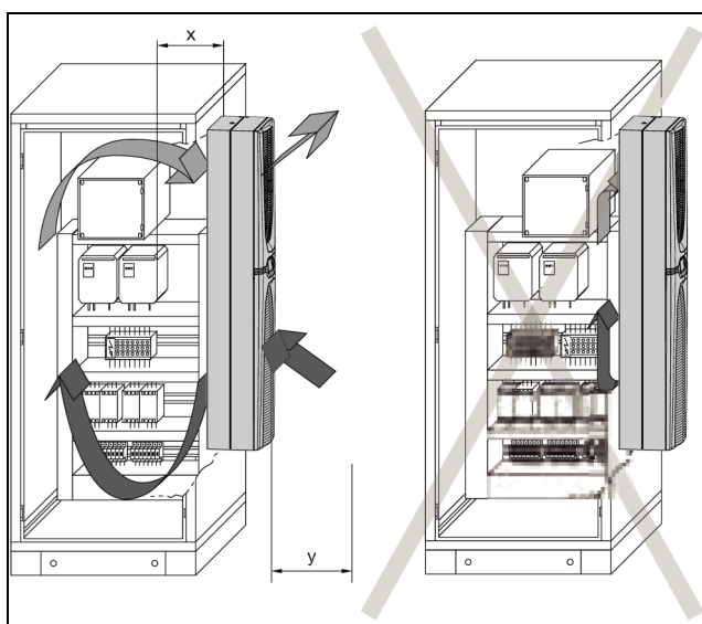
Rys. 5: Cykulacja powietrza w szafie sterowniczej
