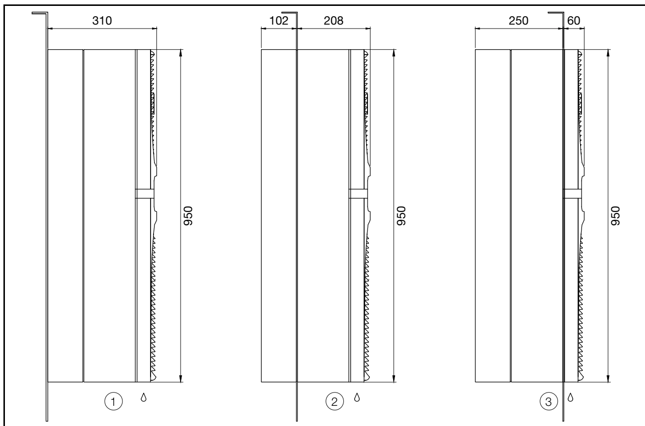
Rys. 41: Wymiary SK 3184837 i SK 3185x3x
