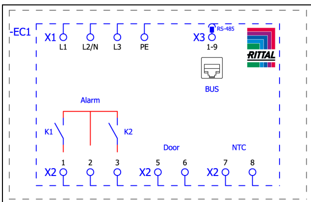
Rys. 17: Schemat połączeń SK 3184837, SK 3185x3x, SK 3186x3x i SK 3187x3x
