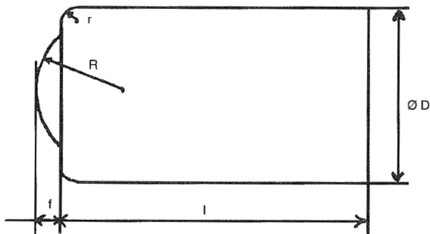
插图1：试验工具的尺寸
