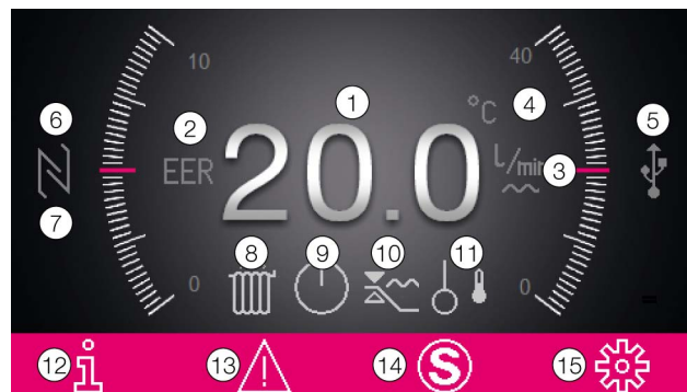
Fig. 44 : structure de l'écran de démarrage
