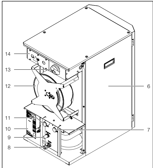
Fig. 13 : vue arrière (sans couvercle)
