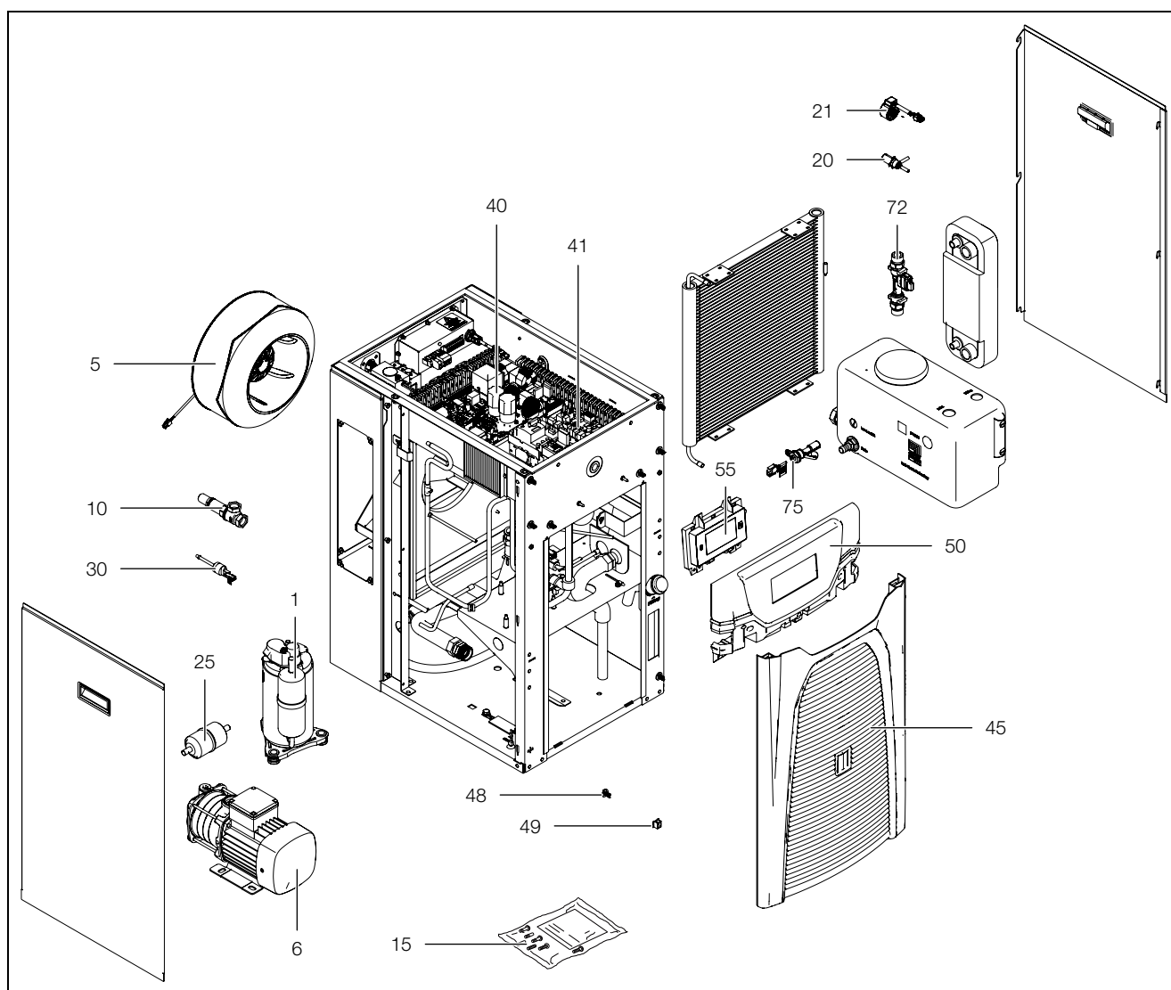
Fig. 62 : pièces détachées
