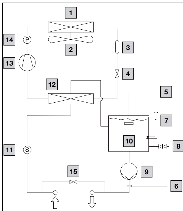
Fig. 9 : schéma fonctionnel du circuit frigorifique
