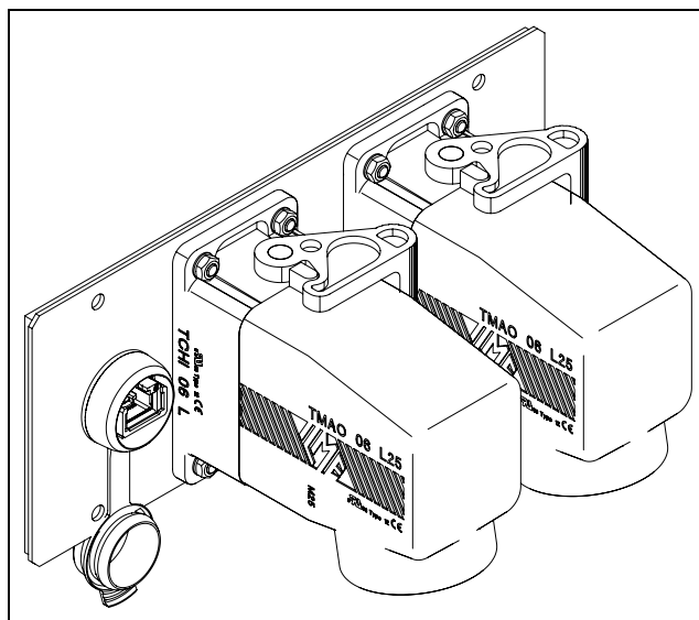
Fig. 26 : prises industrielles
