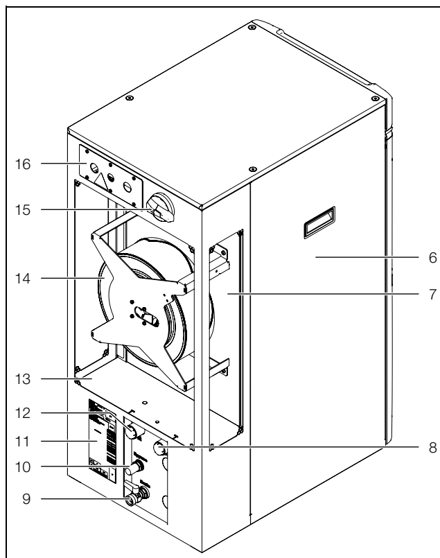
Fig. 4 : vue arrière (3334400)
