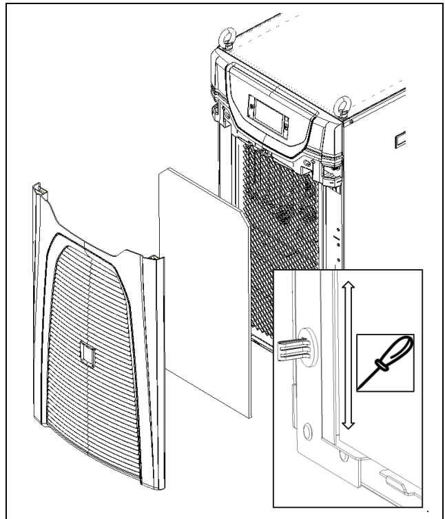
Fig. 35 : installation d'une cartouche filtrante textile 3319100, 3320200 et 3334300
