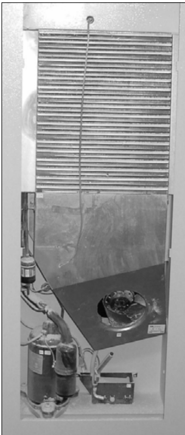
Fig. 29: Modulo unità clima
