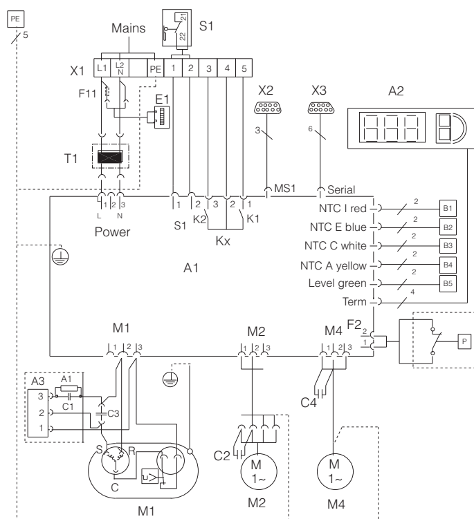
Fig. 21: Schema degli allacciamenti elettrici nr. 1
