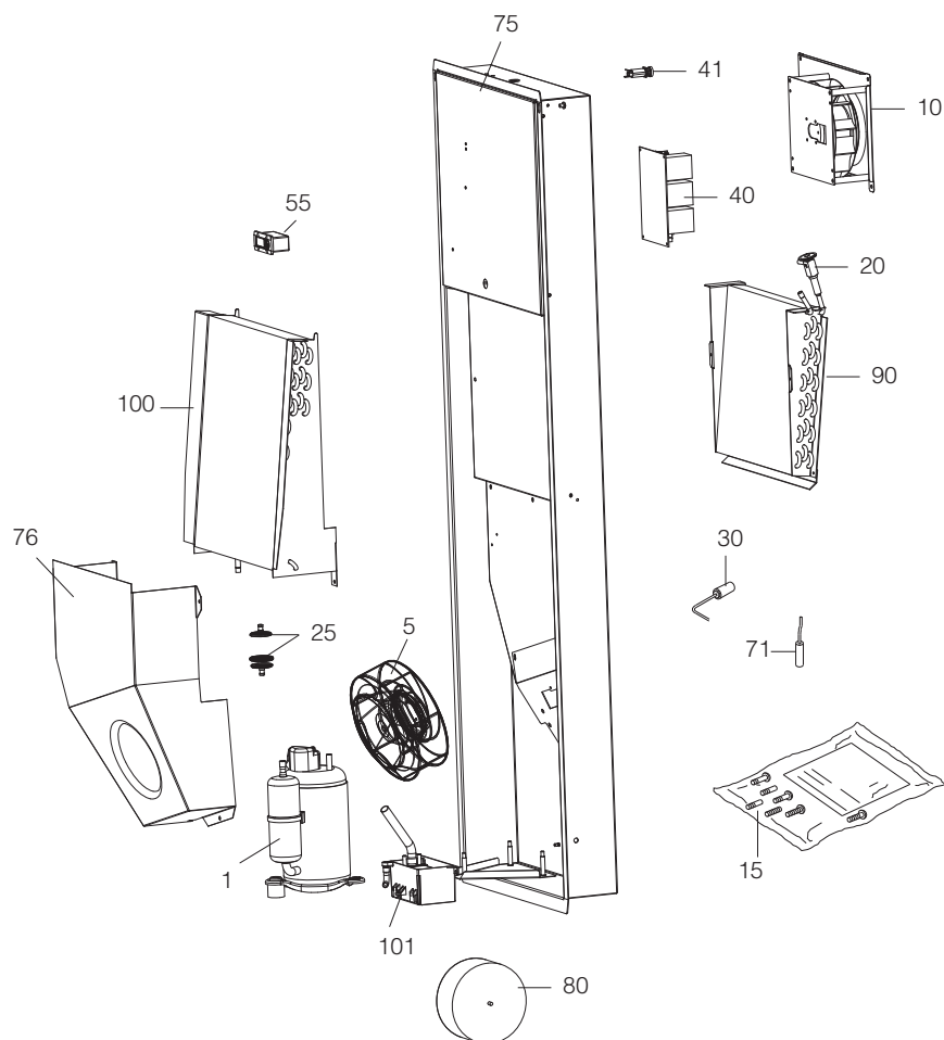
Fig. 32: Parti di ricambio SK 3307.xxx e SK 3310.xxx
