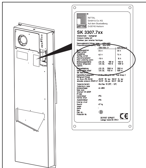
Fig. 31: Targhetta identificativa (dati tecnici)
