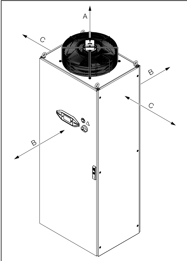
Obr. 7: Minimální vzdálenosti
