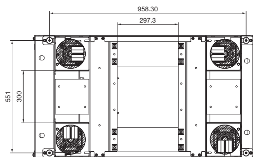
Untersicht
