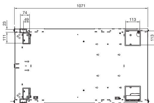
Draufsicht
