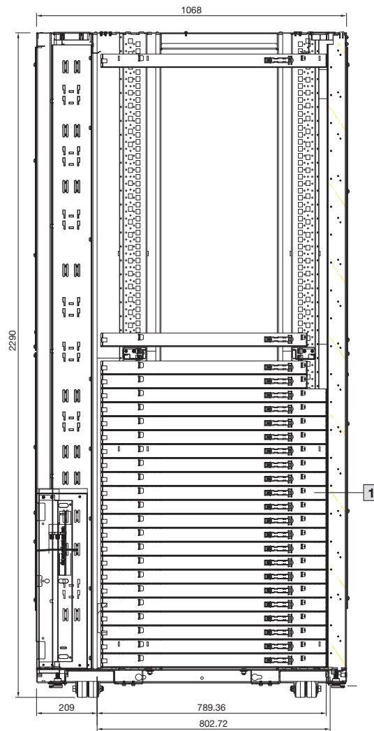
Seitenansicht
