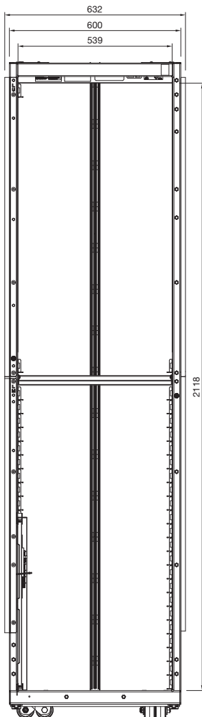
Vorderansicht
