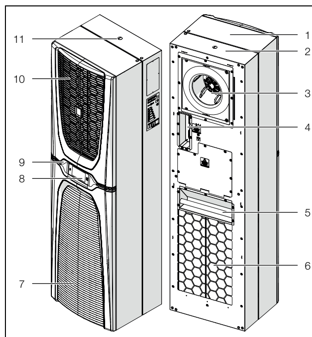
Abb. 2: Hauptkomponenten des Kühlgeräts
