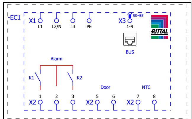
Abb. 17: Schaltplan SK 3484837, SK 3485x3x, SK 3486x3x und SK 3487x3x
