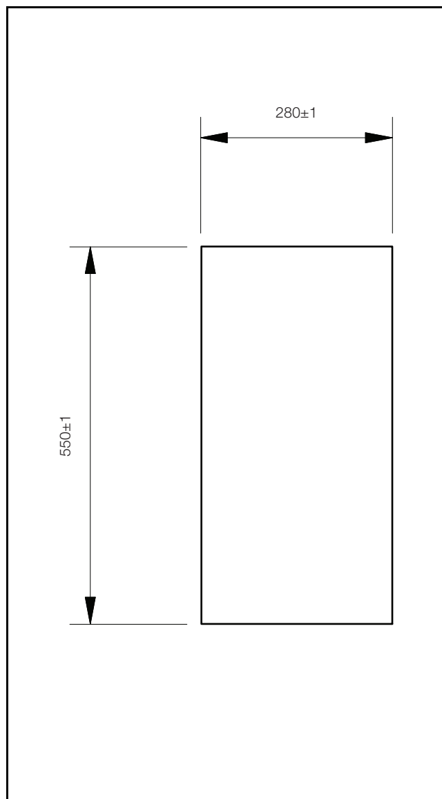
Obr. 65: Wycięcie montażowe
