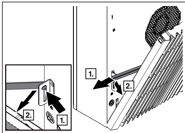
Obr. 26: Odłączanie ograniczników
