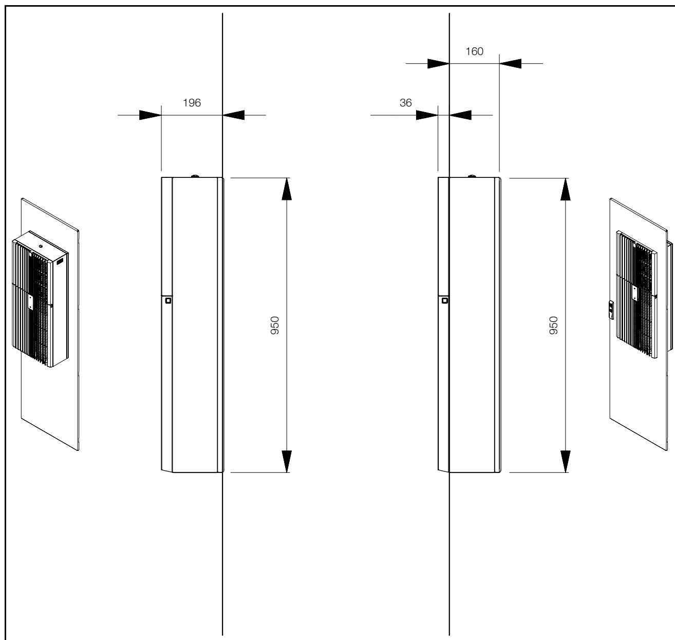
Obr. 70: Wymiary
