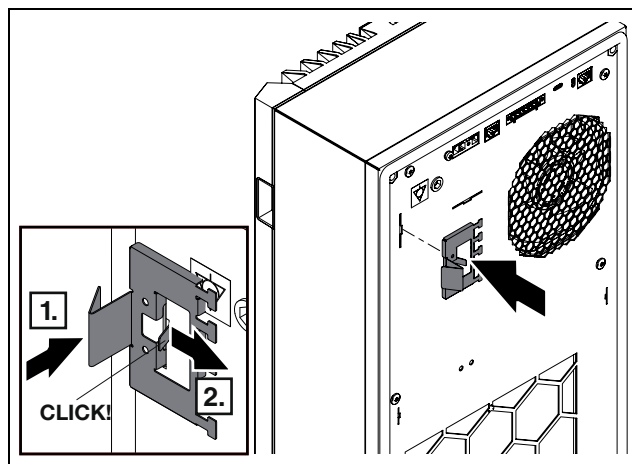
Obr. 11: Zakładanie klamry do podwieszania (dla SK 347880x, SK 347980x i SK 3480800)
