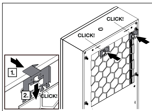
Obr. 31: Zatrzasknięcie klamry do podwieszania (dla SK 34848x0)
