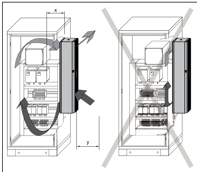
Obr. 7: Cykulacja powietrza w szafie sterowniczej
