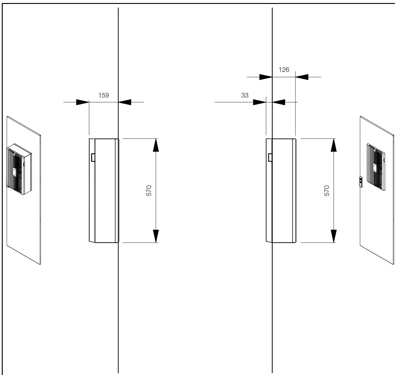
Obr. 67: Wymiary
