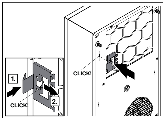
Obr. 30: Zatrzasknięcie klamry do podwieszania (dla SK 347880x, SK 347980x i SK 3480800)
