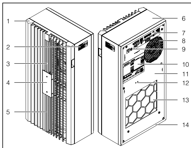
Rys. 2: Główne komponenty klimatyzatora (SK 347880x/SK 347980x/SK 3480800)
