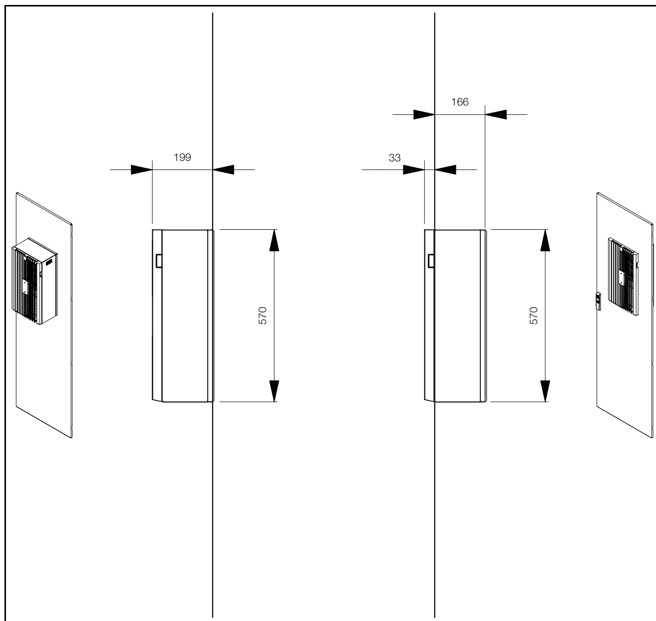
Obr. 68: Wymiary
