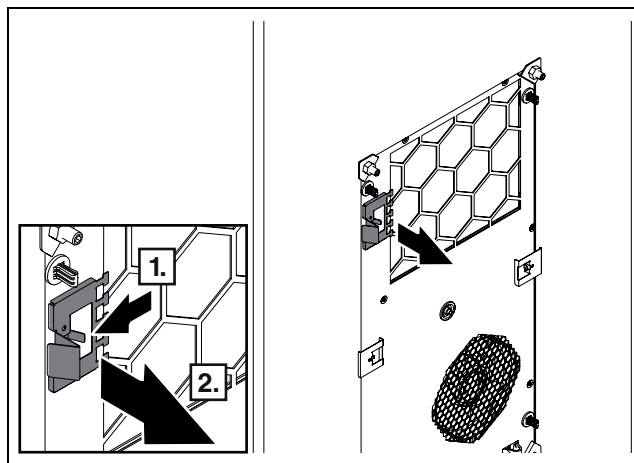
Obr. 40: Odłączanie klamry do podwieszania (dla SK 347880x, SK 347980x i SK 3480800)
