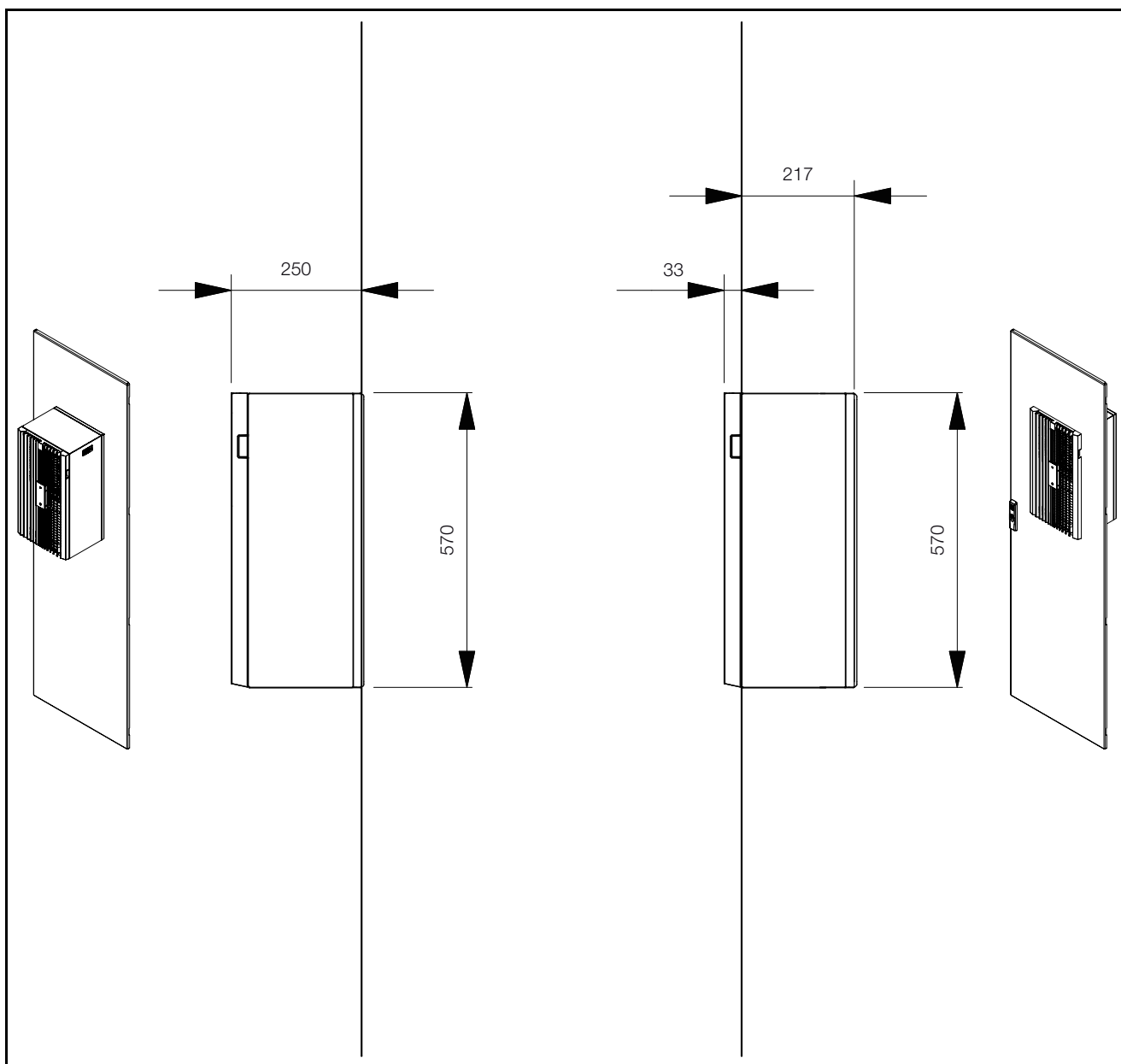
Obr. 69: Wymiary
