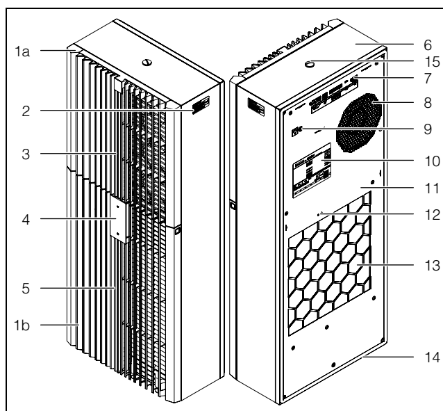
Rys. 3: Główne komponenty klimatyzatora (SK 34848x0)
