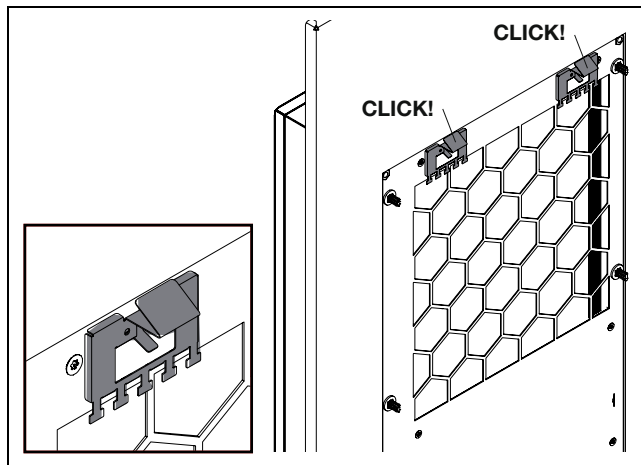
Obr. 35: Zatrzaśnięcie klamry za wycięciem (dla SK 34848x0)
