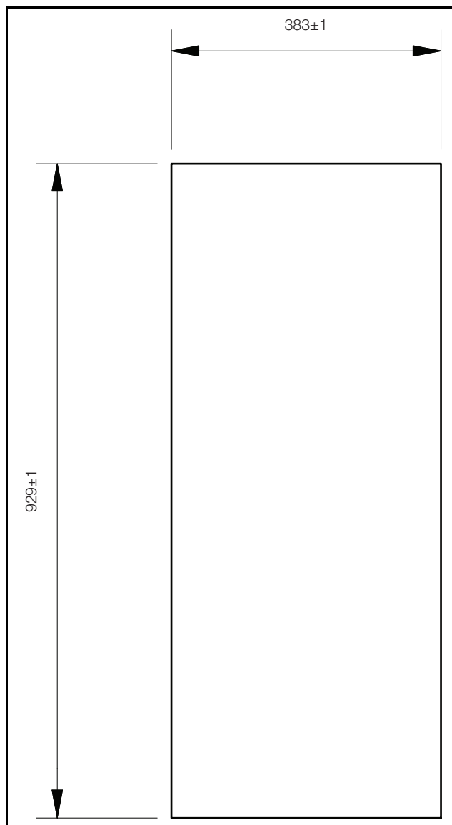
Obr. 66: Wycięcie montażowe
