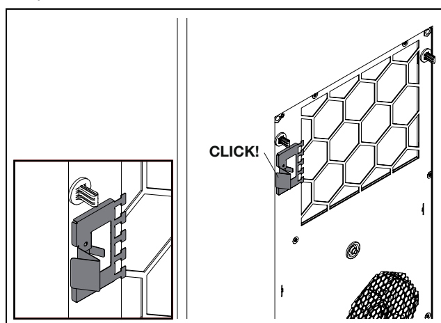
Obr. 34: Zatrzasknięcie klamry za wycięciem (dla SK 347880x, SK 347980x i SK 3480800)
