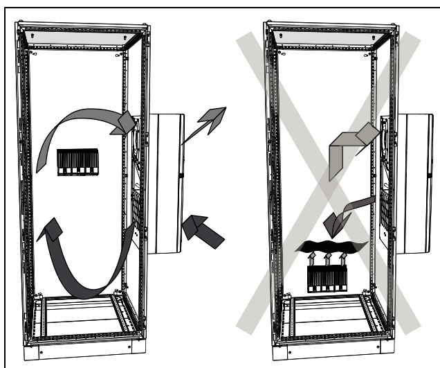
Fig. 6 : ne jamais diriger le flux d'air froid vers des composants actifs (exemple de représentation)
