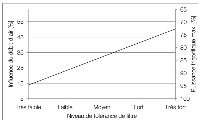
Fig. 24 : exemple de tracé de la puissance frigorifique
