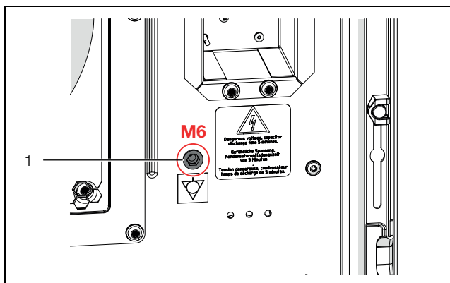
Fig. 15 : point de raccordement pour l'équipotentialité (exemple de représentation)
