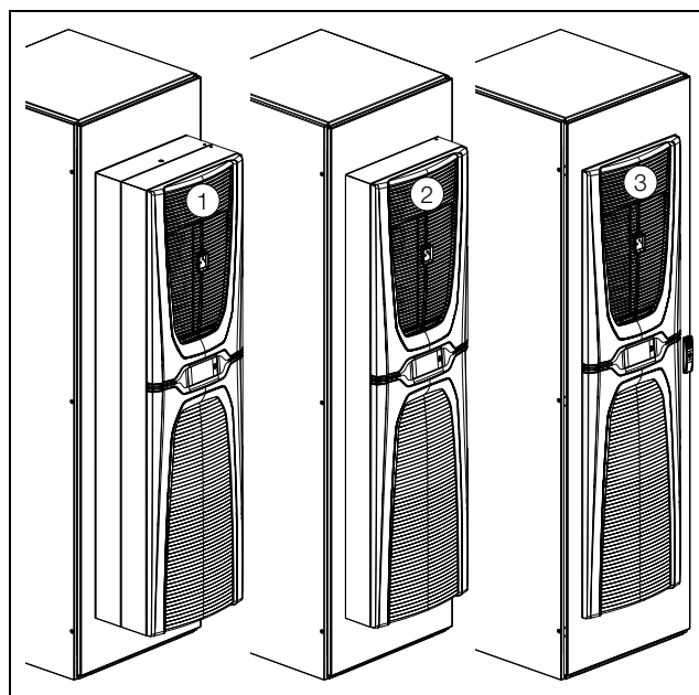
Fig. 7 : possibilités de montage (exemple de représentation)
