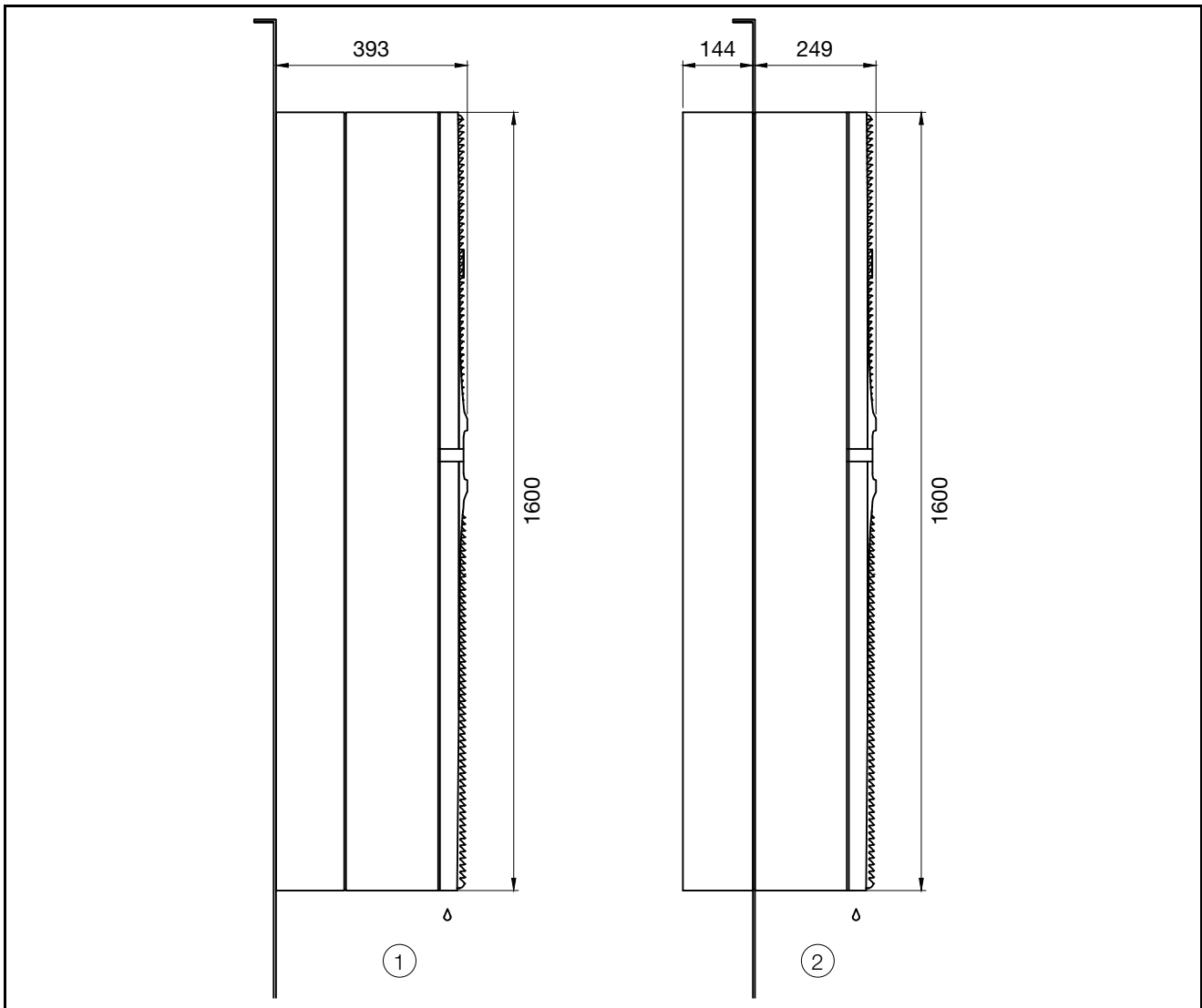
Fig. 42 : dimensions références SK 3488x4x et SK 3489x4x
