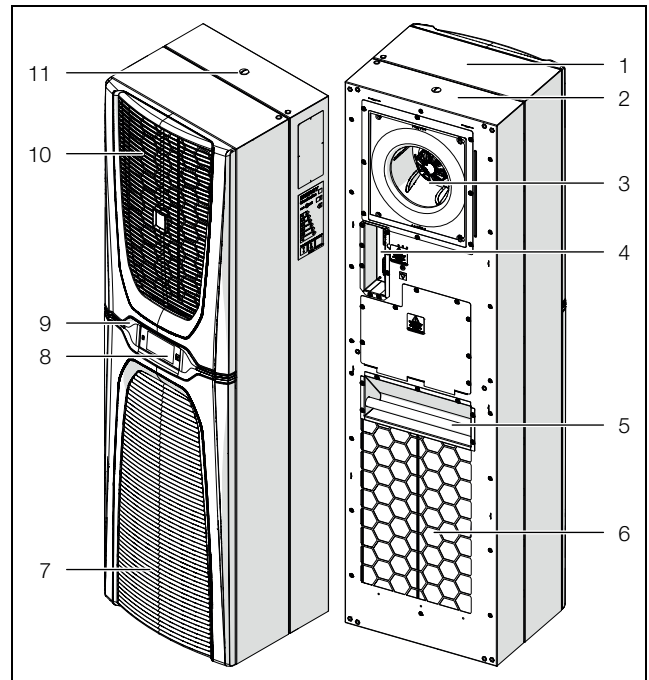
Fig. 2 : composants principaux du climatiseur
