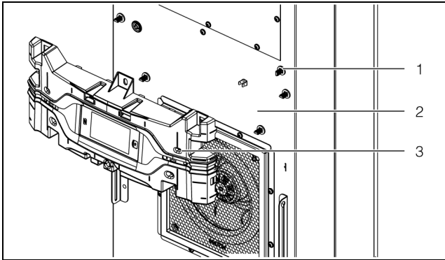
Fig. 31 : enlèvement du bandeau central (exemple de représentation)
