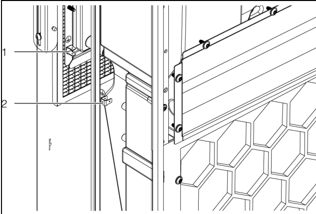
Fig. 35 : raccordement de mise à la masse (vue arrière) (exemple de représentation)
