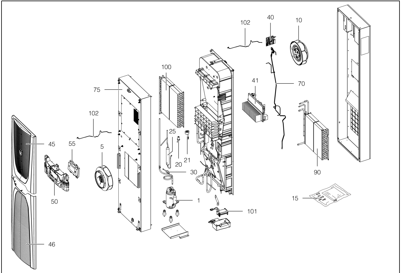
Fig. 36 : pièces de rechange (exemple de représentation)
