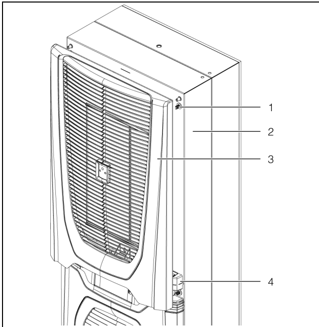
Fig. 28 : ôter la grille à lamelles supérieure (exemple de représentation)
