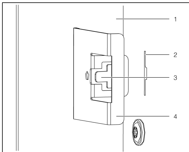
Fig. 34: Allentamento delle clip di fissaggio
