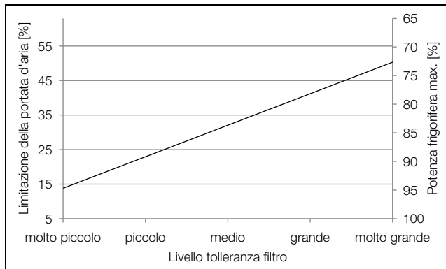
Fig. 24: Esempio di andamento della potenza frigorifera
