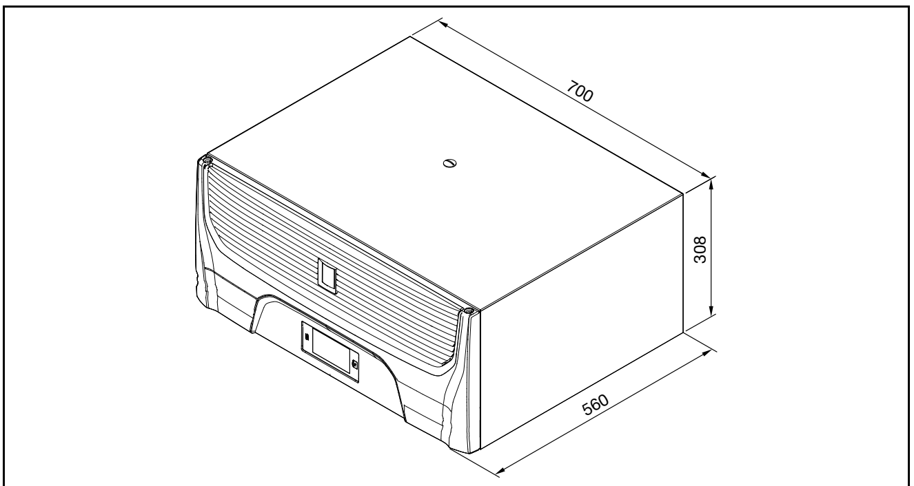
Abb. 23: Abmessungen
