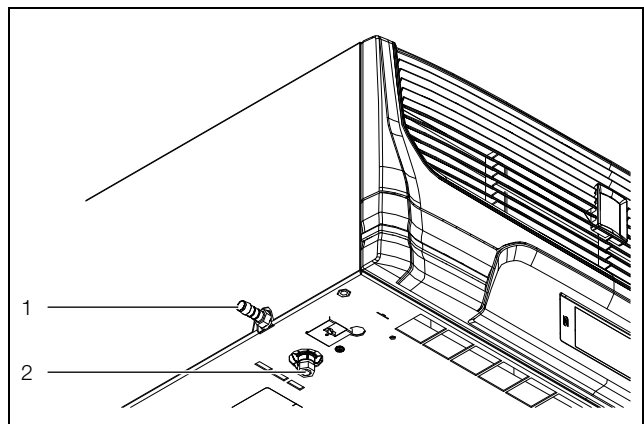
Abb. 6: Anschluss für Kondensatwasserablaufschlauch
