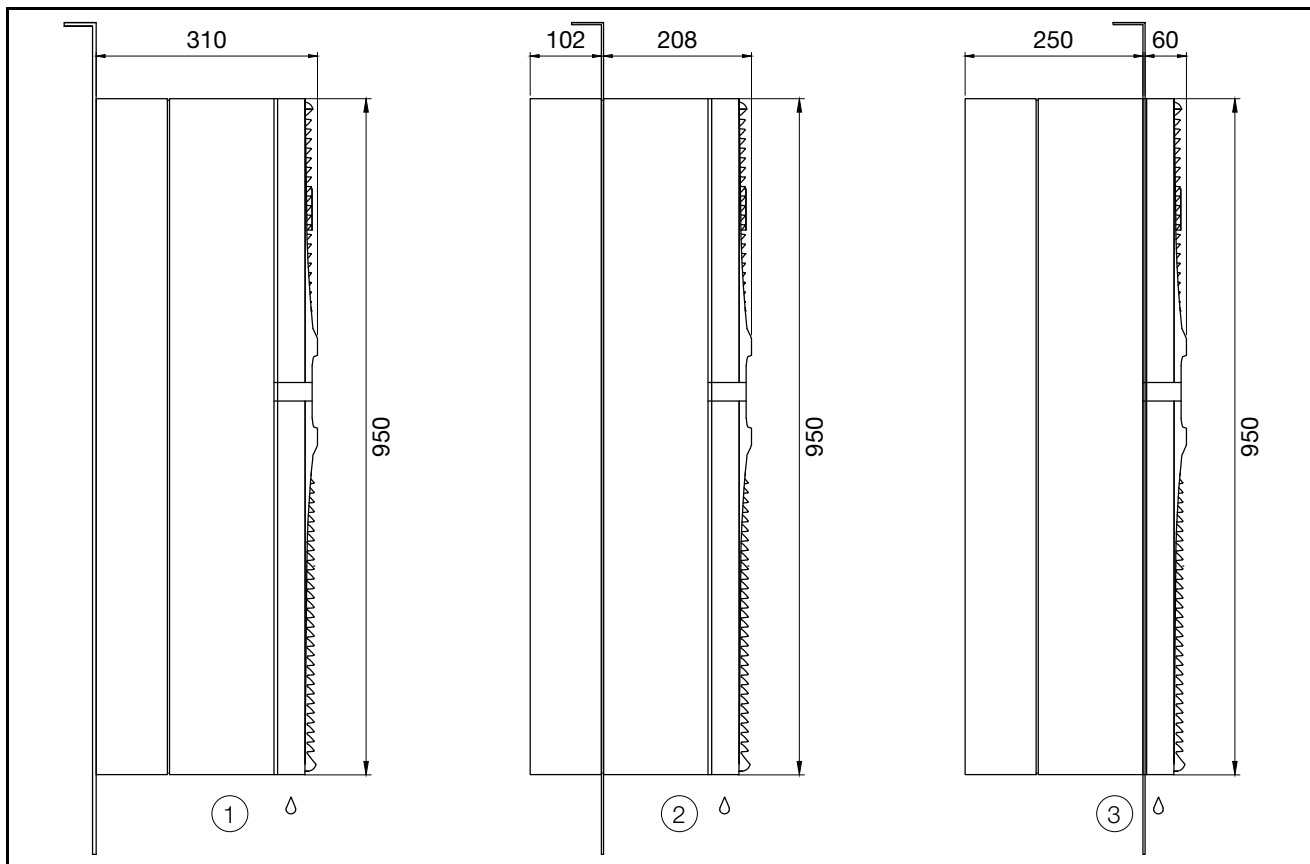
Rys. 40: Wymiary SK 3484837 i SK 3485x3x
