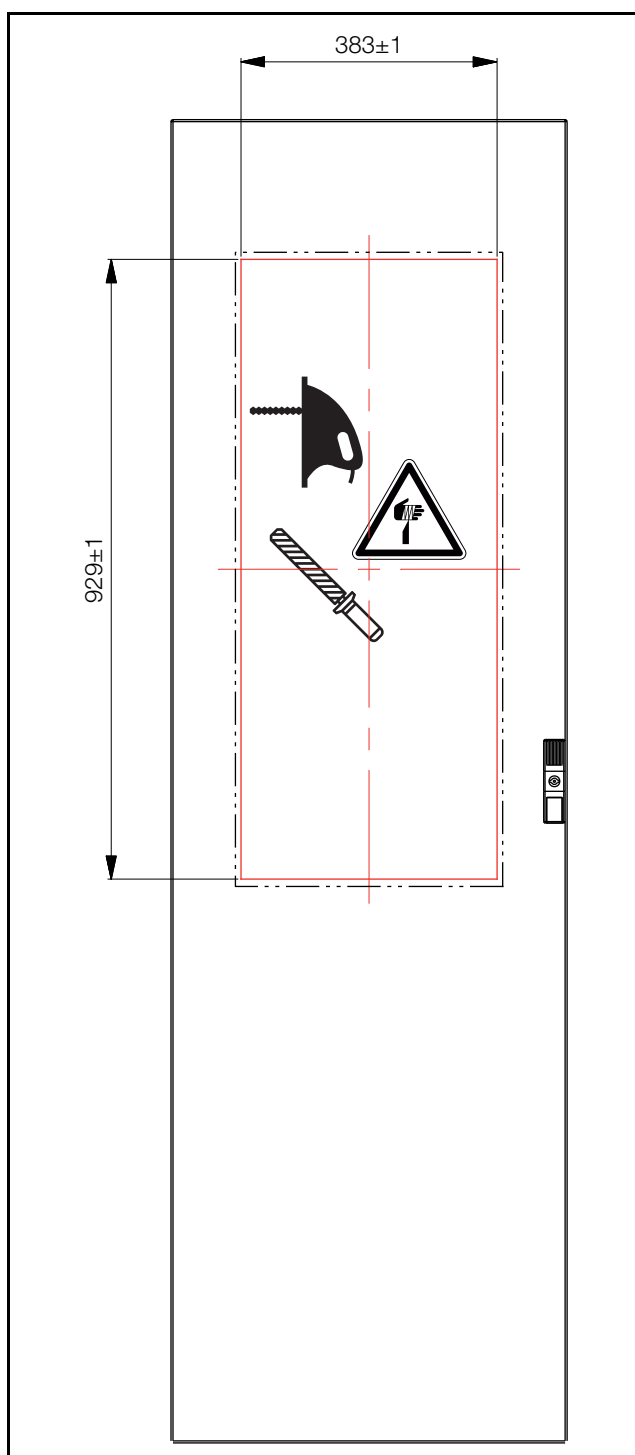
Rys. 37: Wycięcie montażowe
