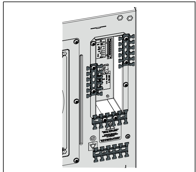
Rys. 19: Instalacja szyny do prowadzenia kabli (przykładowa ilustracja)
