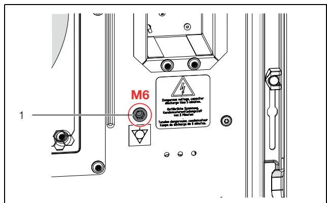
Rys. 15: Złącze wyrównania potencjałów (przykładowa ilustracja)
