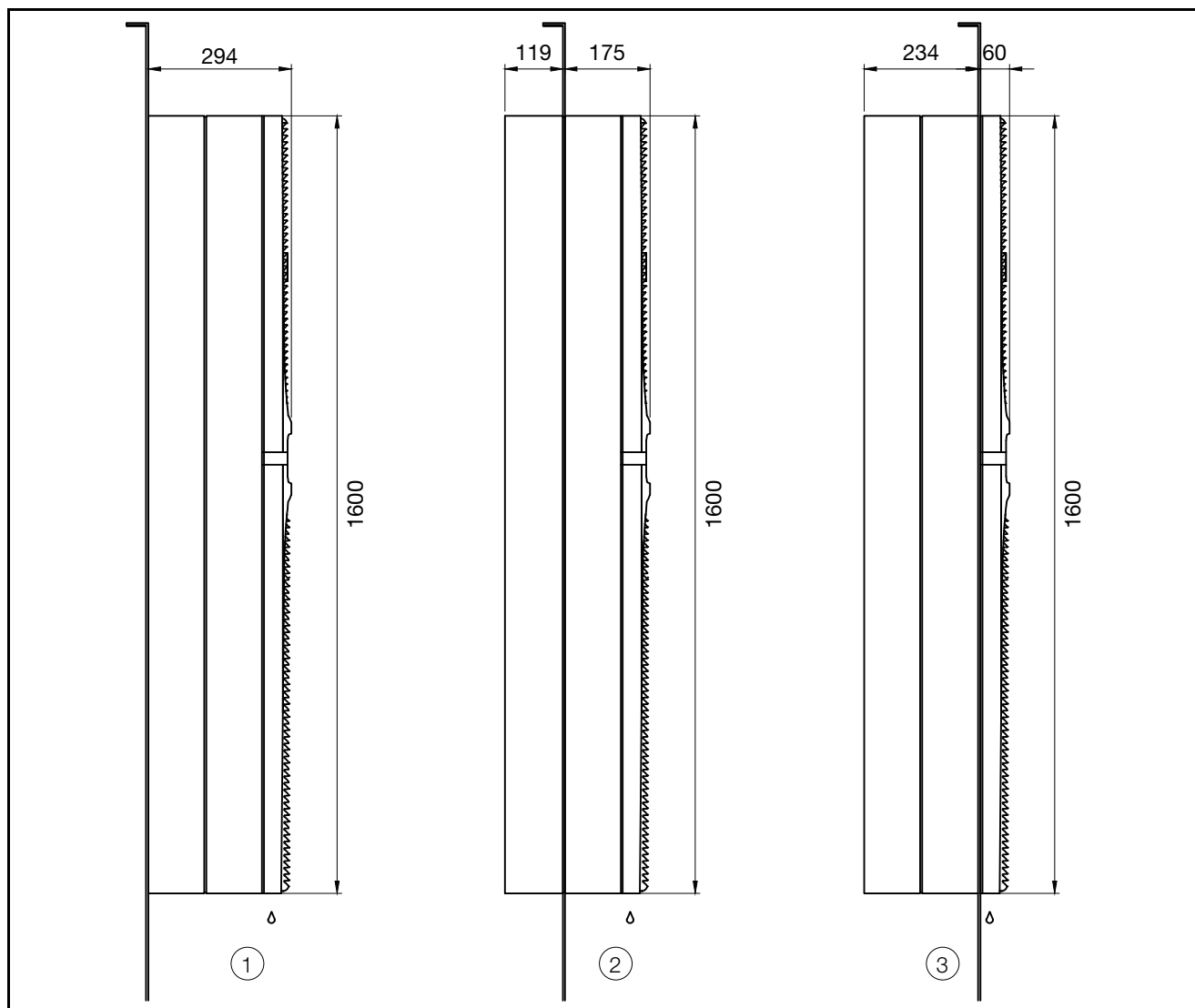
Rys. 41: Wymiary SK 3486x3x i SK 3487x3x
