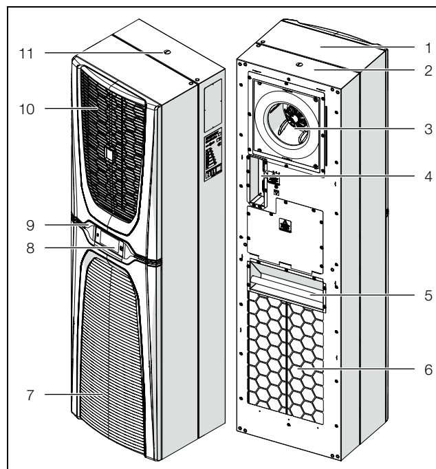
Rys. 2: Główne komponenty klimatyzatora
