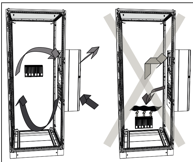
Rys. 6: Nigdy nie kierować strumienia zimnego powietrza na aktywne komponenty (przykładowa ilustracja)
