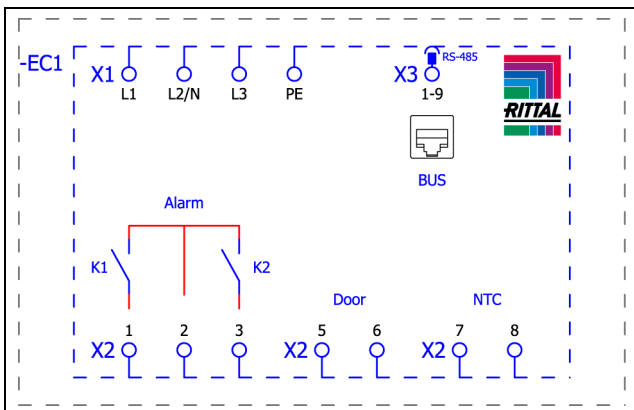
Rys. 17: Schemat połączeń SK 3484837, SK 3485x3x, SK 3486x3x i SK 3487x3x
