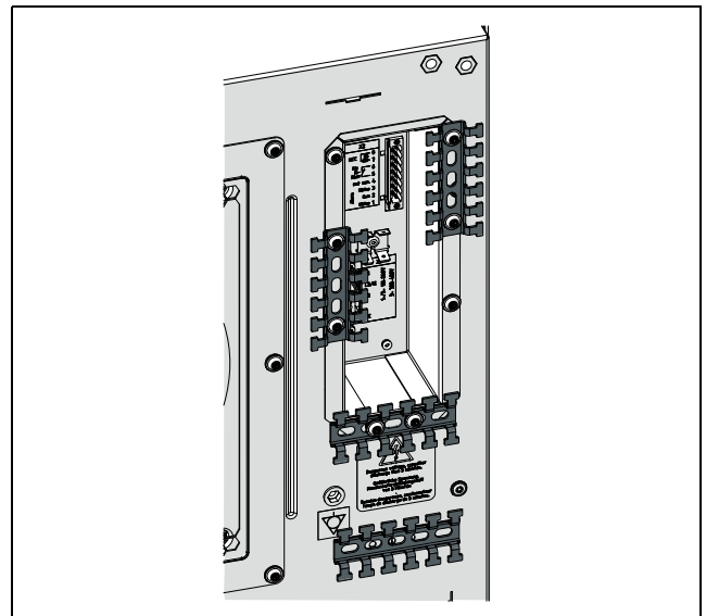
Fig. 19: Montagem da guia para cabos (exemplo)
