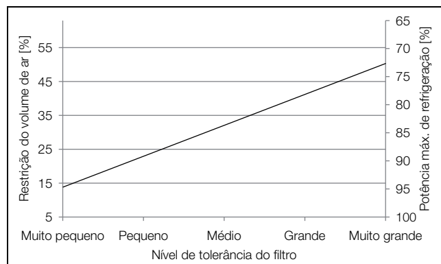
Fig. 24: Exemplo de progressão da potência de refrigeração
