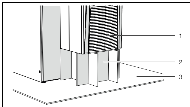
Fig. 4: Material para transporte com segurança
