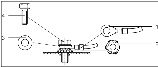
Fig. 16: Instalação da ligação equipotencial
