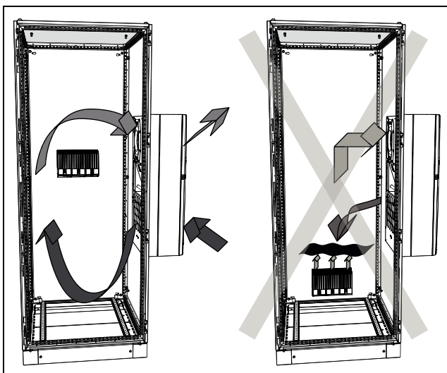
Fig. 6: Nunca direcionar a corrente de ar frio para os componentes ativos (exemplo)
