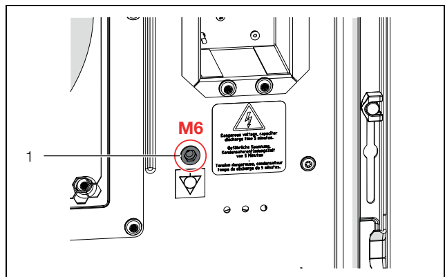
Fig. 15: Ponto de conexão da ligação equipotencial (exemplo)
