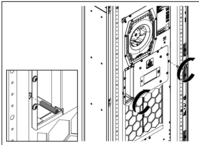
Fig. 16 : vissage des tiges filetées du milieu
