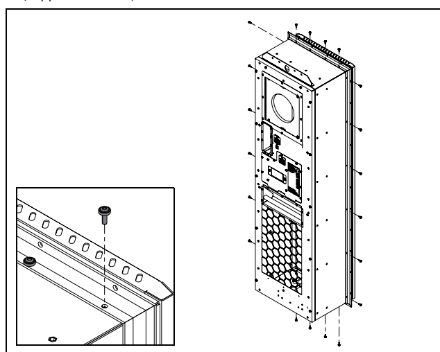
Fig. 23 : fixation du cadre de montage sur le climatiseur
