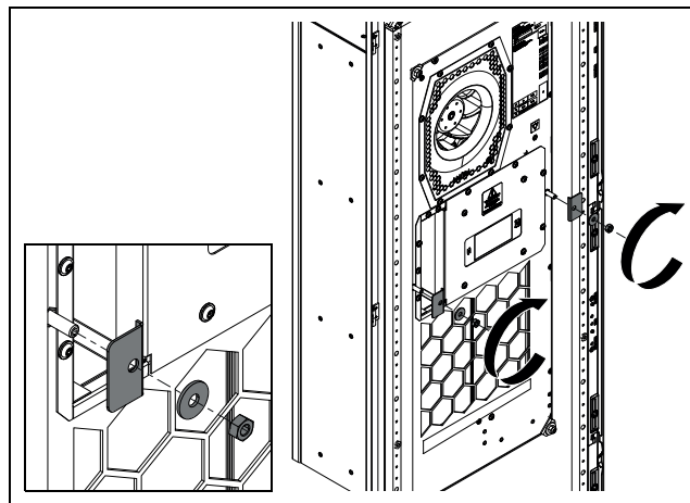
Fig. 18 : montage des équerres en L du milieu
