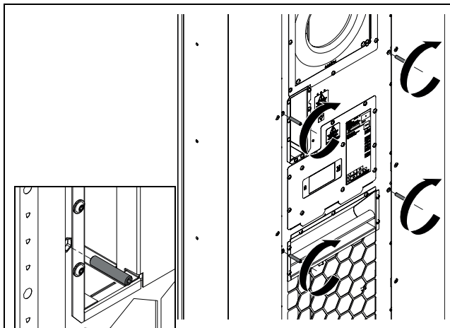
Fig. 17 : vissage des tiges filetées du milieu
