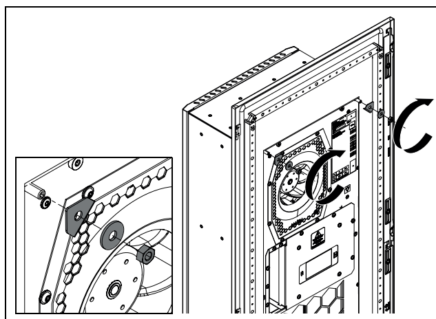
Fig. 14 : montage des équerres d'angle supérieures
