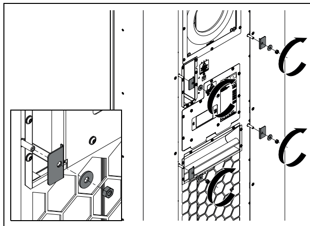
Fig. 19 : montage des équerres en L du milieu
