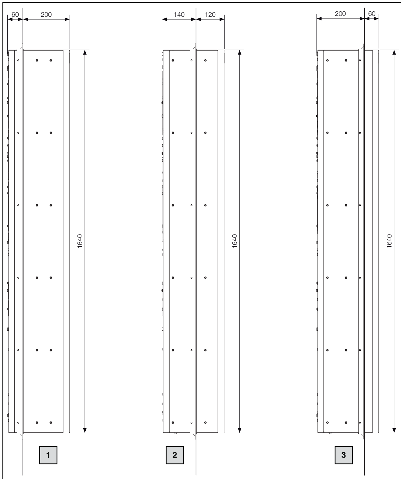
Fig. 54 : dimensions
