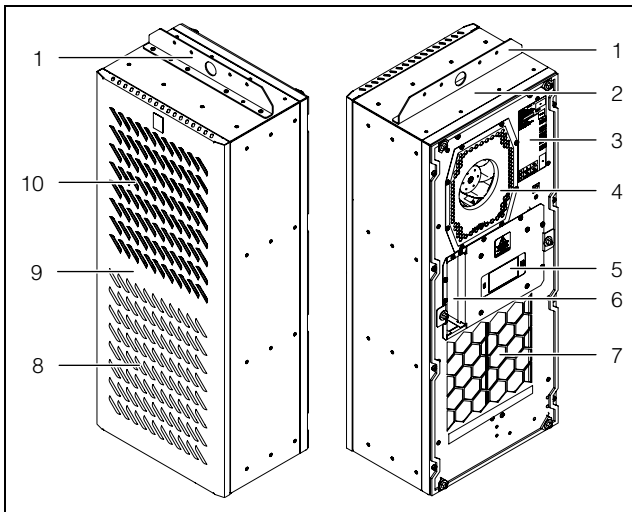
Fig. 2 : composants principaux du climatiseur (référence SK 3485330)
