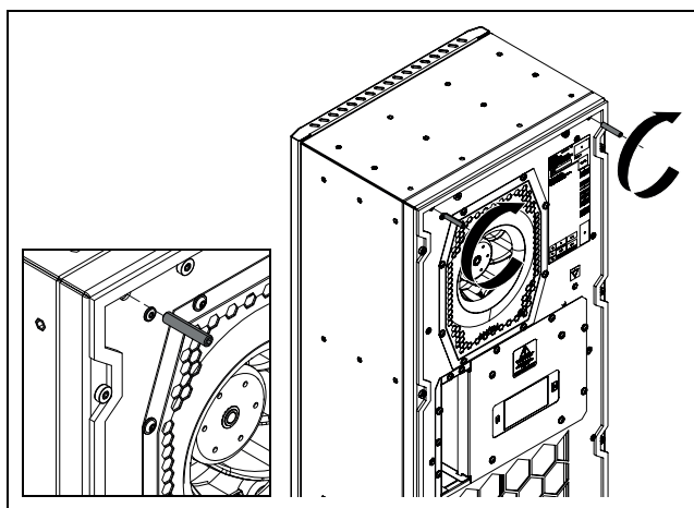
Fig. 12 : vissage des tiges filetées supérieures
