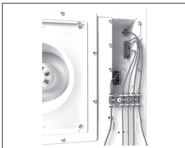
Fig. 40 : réalisation de la décharge de traction à l'aide de colliers de câblage (exemple d'illustration)
