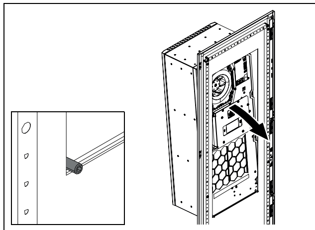
Fig. 13 : pose du climatiseur dans la découpe de montage
