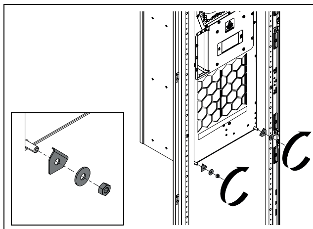
Fig. 15 : montage des équerres d'angle inférieures
