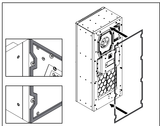
Fig. 10 : pose du joint
