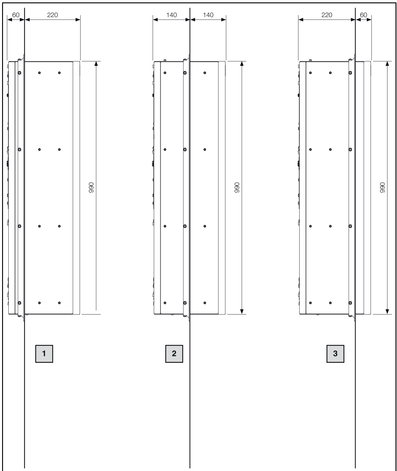
Fig. 53 : dimensions
