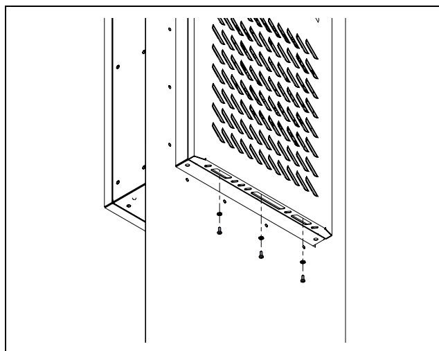
Fig. 47: Allentamento delle viti di fissaggio
