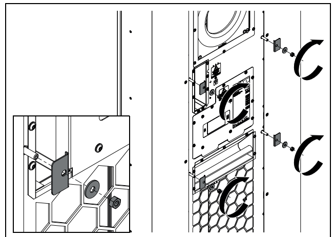
Fig. 19: Montaggio degli angolari a L centrali
