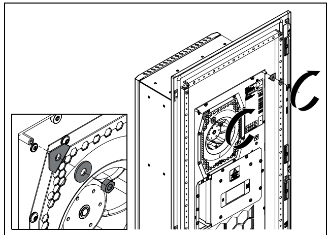
Fig. 14: Montaggio degli angolari superiori
