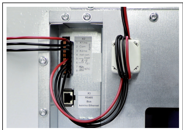
Fig. 32: Punto di montaggio del nucleo di ferrite in SK 3485330
