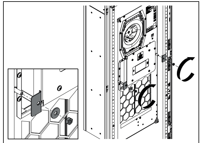
Fig. 18: Montaggio degli angolari a L centrali
