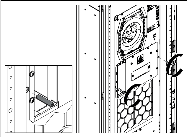
Fig. 16: Avvitamento dei perni filettati centrali
