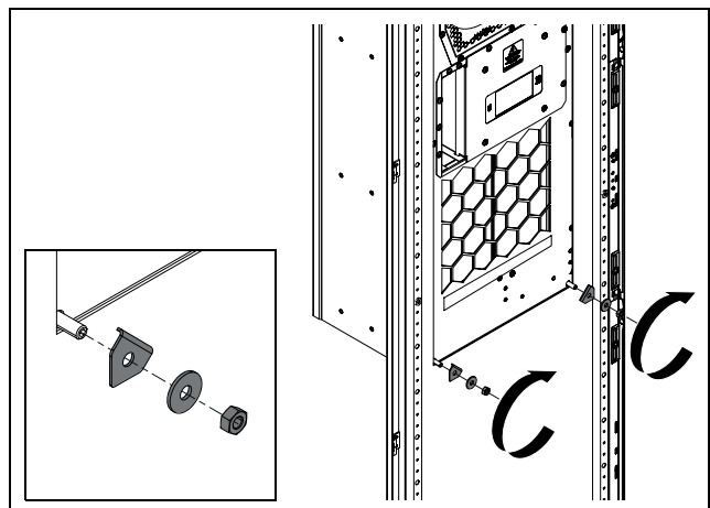
Fig. 15: Montaggio degli angolari inferiori
