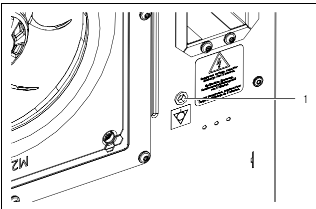
Fig. 34: Punto di collegamento equipotenziale (figura a titolo d'esempio)
