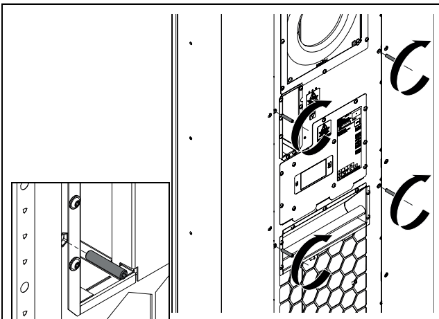
Fig. 17: Avvitamento dei perni filettati centrali
