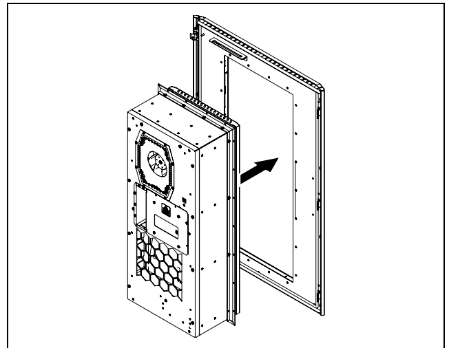
Fig. 26: Inserimento del condizionatore in una parte piana a doppia parete
