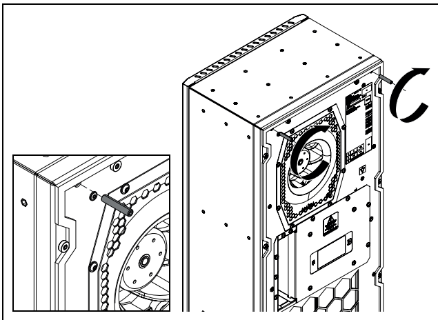
Rys. 12: Wkręcanie górnych trzpieni gwintowanych
