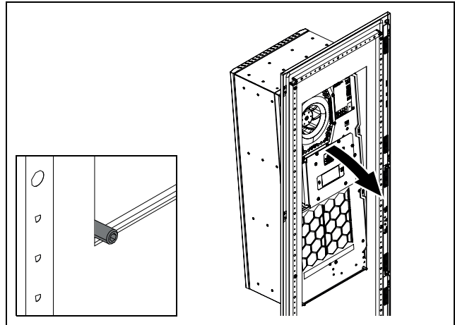
Rys. 13: Osadzanie klimatyzatora w otworze montażowym
