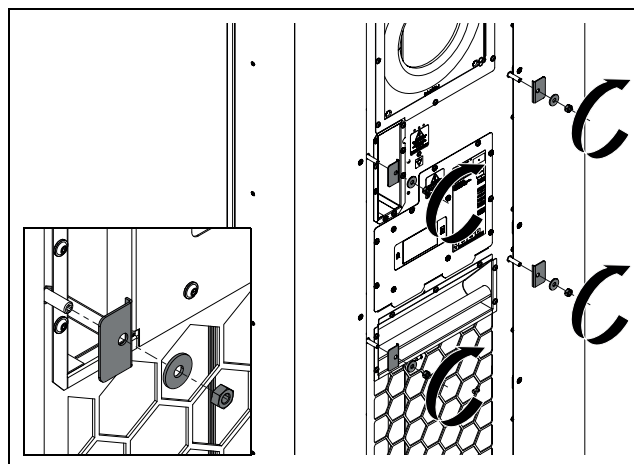
Rys. 19: Montaż środkowych kątowników w kształcie litery L
