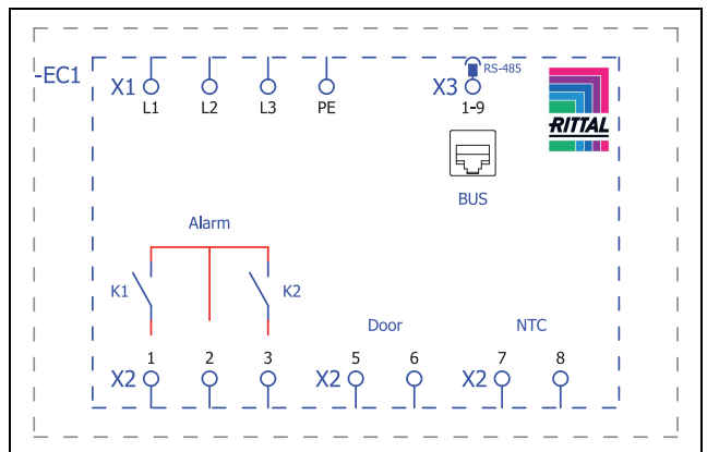
Rys. 38: Schemat połączeń SK 3488340, SK 3489340
