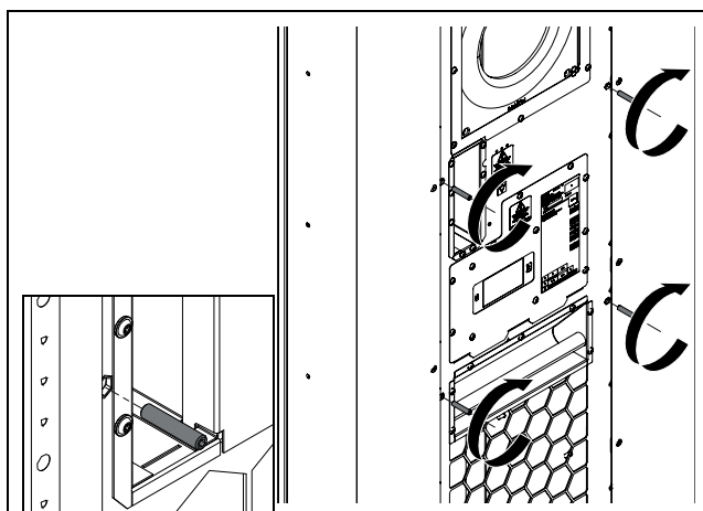
Rys. 17: Wkręcanie środkowych trzpieni gwintowanych
