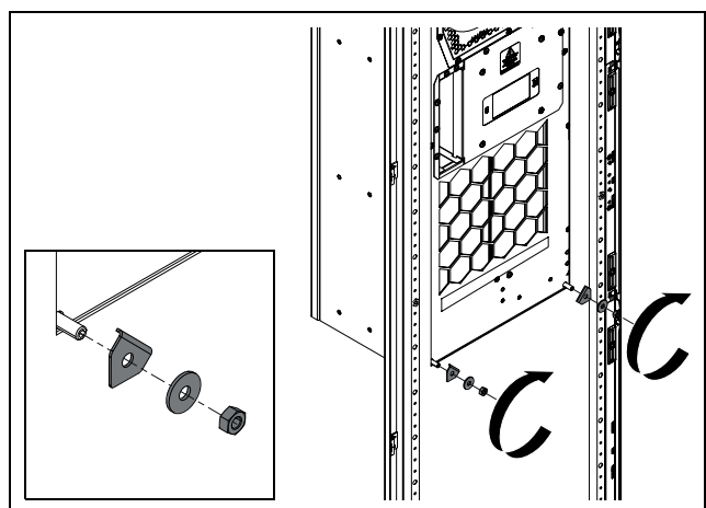
Rys. 15: Montaż dolnych elementów narożnych
