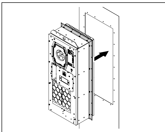
Rys. 25: Osadzanie klimatyzatora w jednościennej części płaskiej
