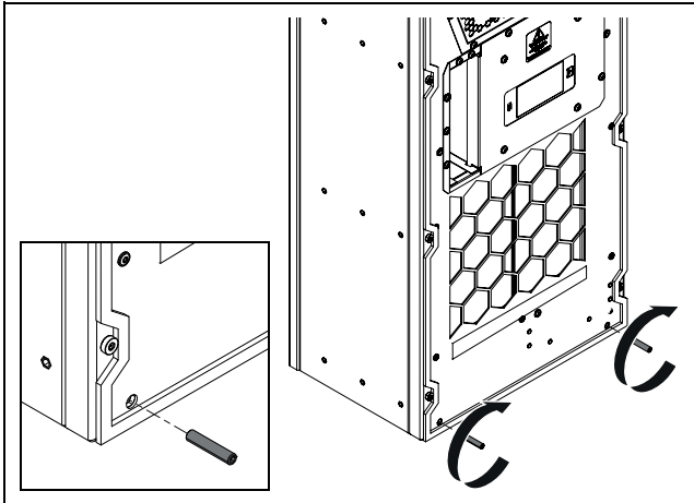
Rys. 11: Wkręcanie dolnych trzpieni gwintowanych
