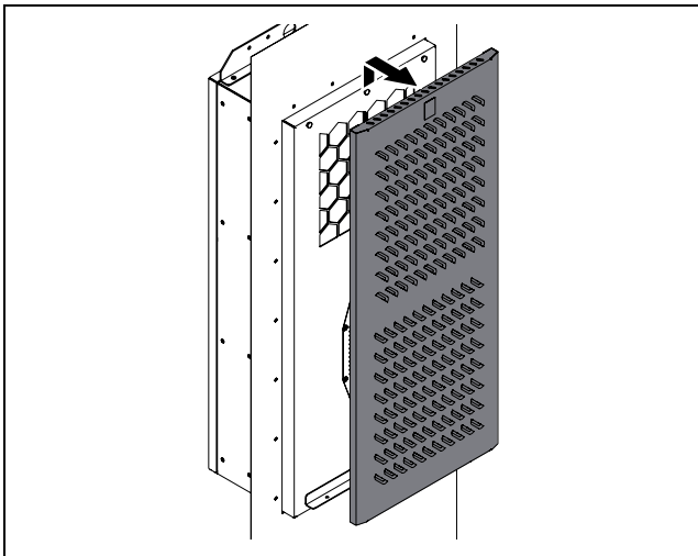
Rys. 28: Podnoszenie osłony
