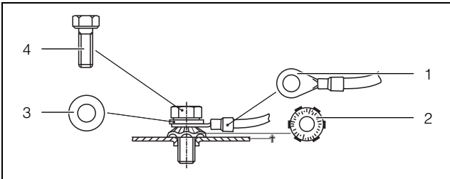
Rys. 35: Wykonanie wyrównania potencjałów
