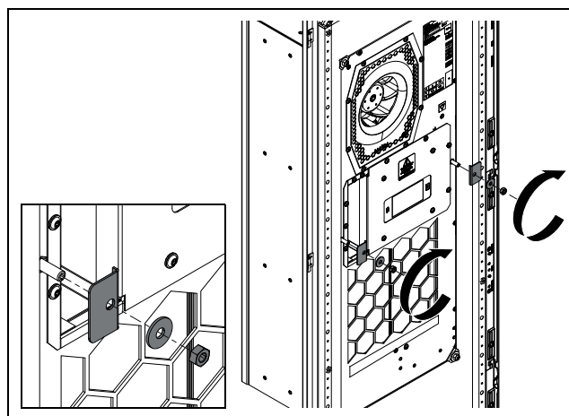
Rys. 18: Montaż środkowych kątowników w kształcie litery L
