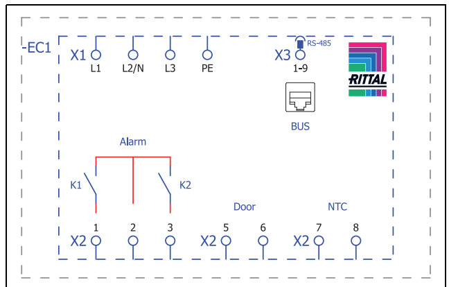
Rys. 37: Schemat połączeń SK 3485330, SK 3486330, SK 3487330
