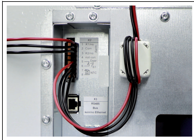
Rys. 32: Punkt montażu rdzenia ferrytowego przy SK 3485330
