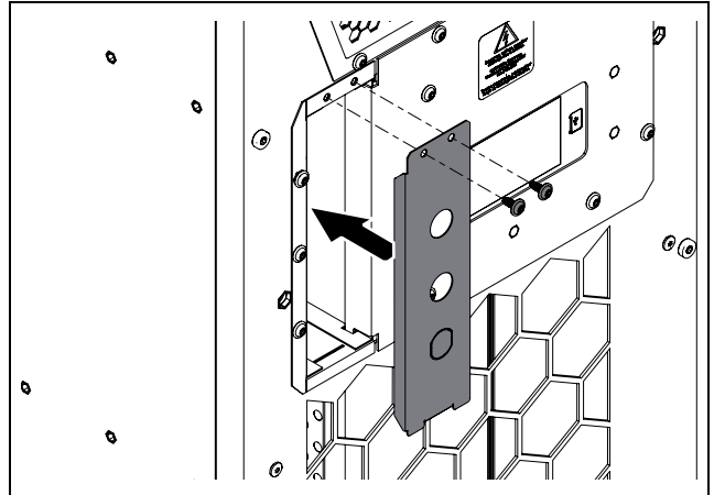
Rys. 36: Montaż pokrywy
