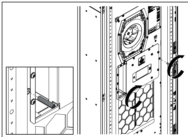
Rys. 16: Wkręcanie środkowych trzpieni gwintowanych
