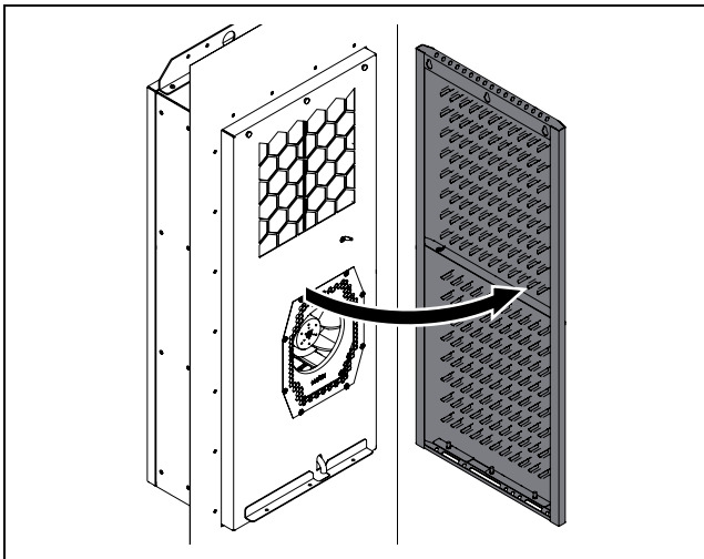
Rys. 29: Odchylanie osłony
