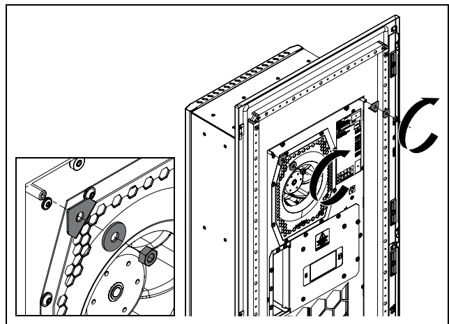
Rys. 14: Montaż górnych elementów narożnych
