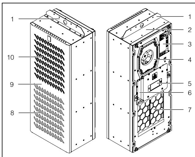
Obr. 2: Hlavní části chladicí jednotky (SK 3485330)
