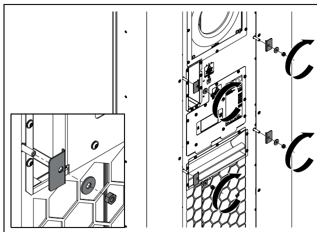
Obr. 19: Montáž prostředních úhelníků ve tvaru L
