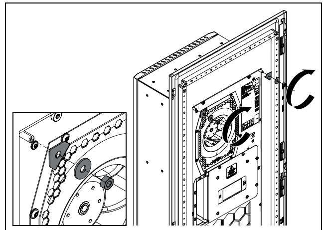
Obr. 14: Montáž horních rohových úhelníků
