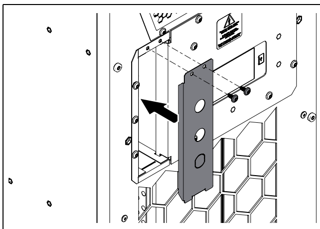
Obr. 36: Montáž krytu
