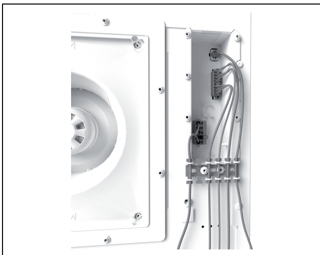
Obr. 40: Odlehčení v tahu pomocí vázacích kabelových pásek (na obrázku je znázorněn příklad)
