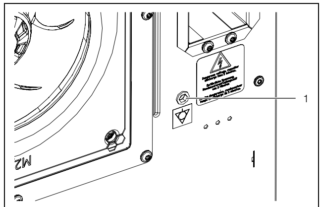
Obr. 34: Připojovací bod pro vyrovnání potenciálů (na obrázku je znázorněn příklad)
