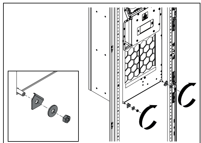
Obr. 15: Montáž dolních rohových úhelníků
