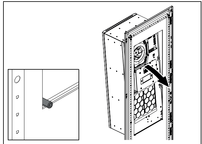
Obr. 13: Usazení chladicí jednotky do montážního výřezu
