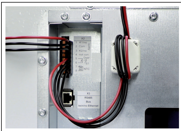
Obr. 32: Upevňovací bod pro feritové jádro na SK 3485330
