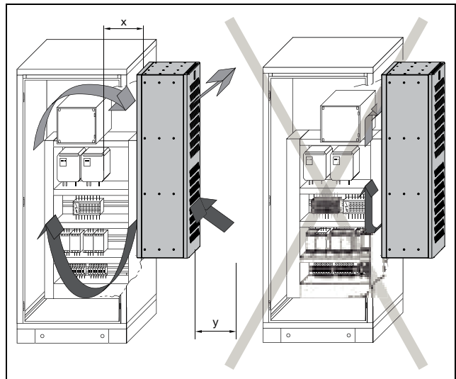
Obr. 6: Cirkulace vzduchu v rozváděčové skříni
