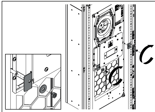
Obr. 18: Montáž prostředních úhelníků ve tvaru L
