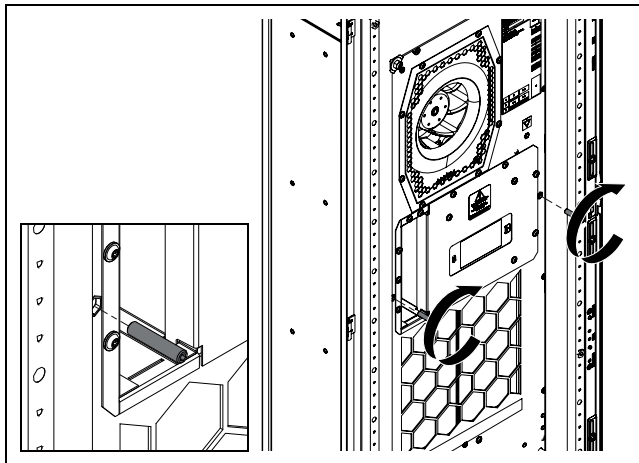
Obr. 16: Zašroubování prostředních závitových svorníků
