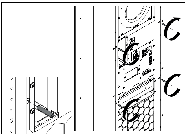
Obr. 17: Zašroubování prostředních závitových svorníků
