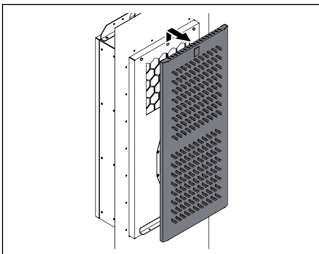
Obr. 28: Zvednutí předního krytu
