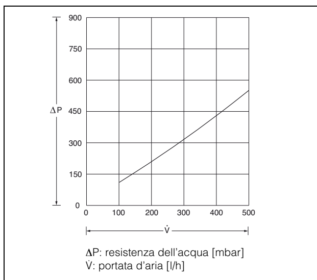
Fig. 35: Resistenza dell'acqua SK 3364.XXX
