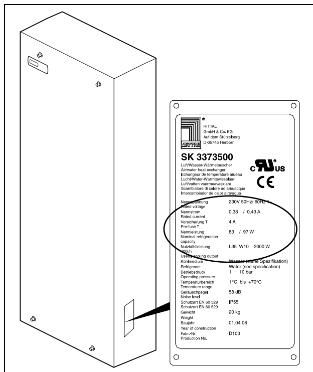
Fig. 31: Targhetta identificativa (dati tecnici)
