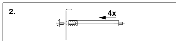
Fig. 11: Fissaggio dei distanziali
