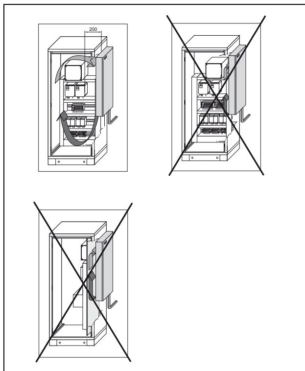
Fig. 4: Conduzione mirata dell'aria all'interno dell'armadio
