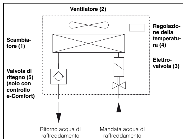
Fig. 2: Scambiatore di calore aria/acqua
