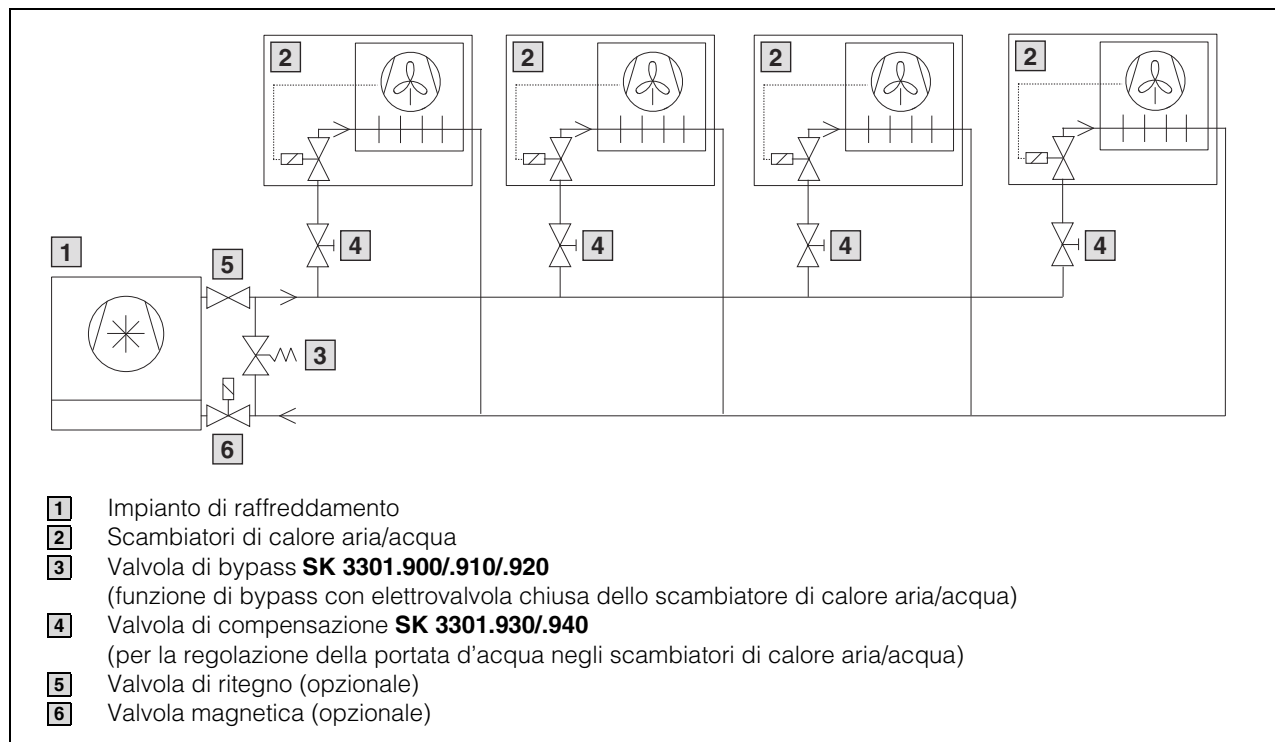
Fig. 42: Collegamento in parallelo di 4 scambiatori di calore aria/acqua
