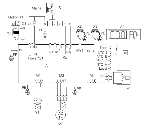
Fig. 18: Schema degli allacciamenti elettrici nr. 2
