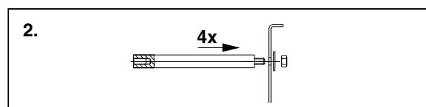
Fig. 6: Inserire e fissare i distanziali nelle apposite forature
