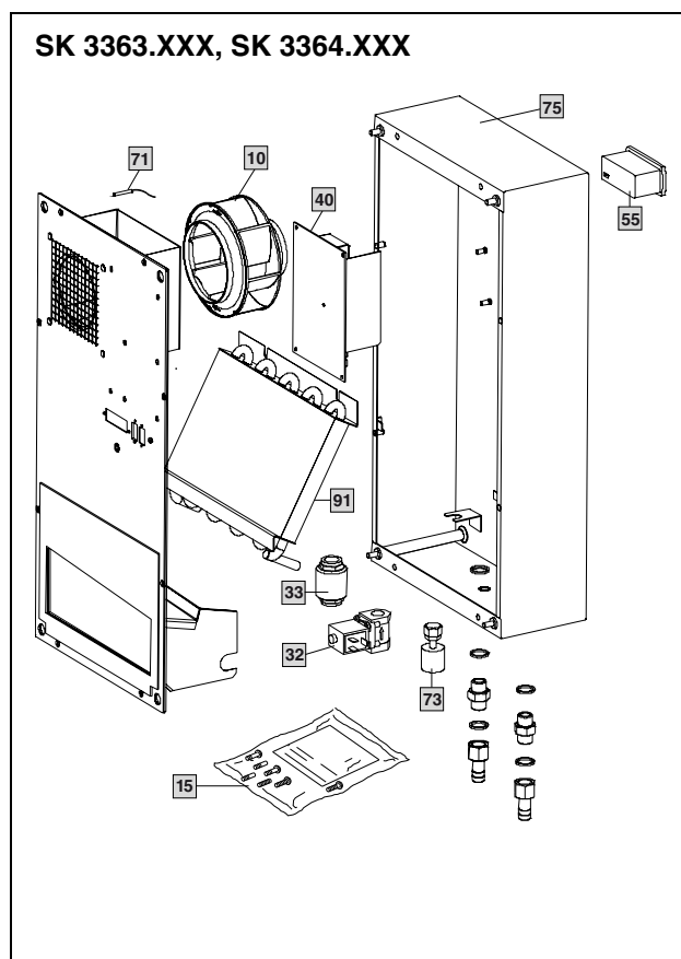
Fig. 32: Parti di ricambio per SK 3363.XXX, SK 3364.XXX
