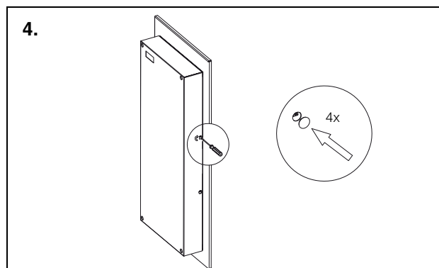
Fig. 13: Chiudere le aperture nella calotta
