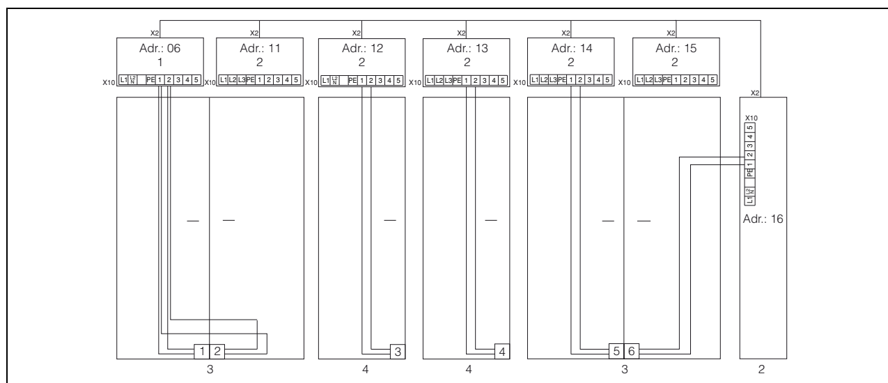
Fig. 24: Esempio di connessione: interruttore di posizione della porta e configurazione master-slave
