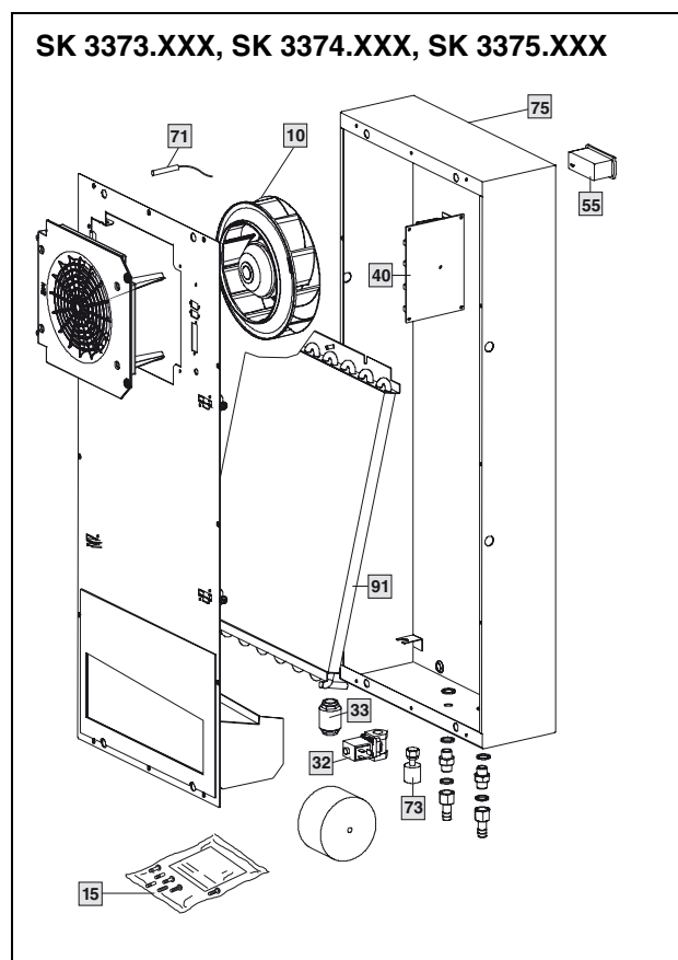
Fig. 33: Parti di ricambio per SK 3373.XXX, SK 3374.XXX, SK 3375.XXX
