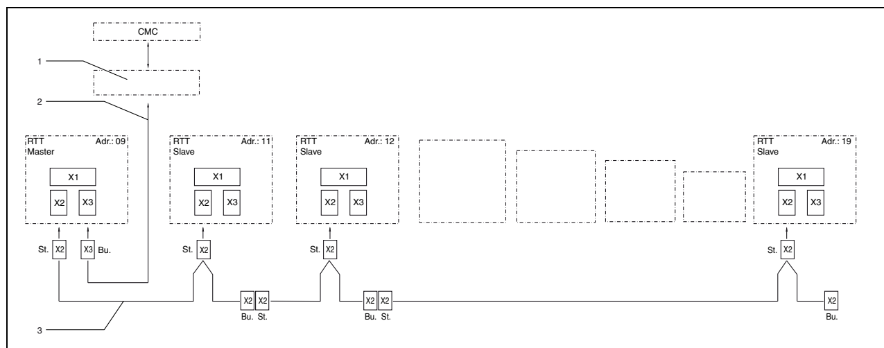
Fig. 23: Esempio di connessione: configurazione master-slave
