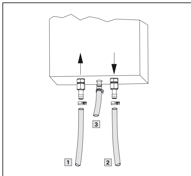
Fig. 15: Raccordi mandata e ritorno acqua di raffreddamento
