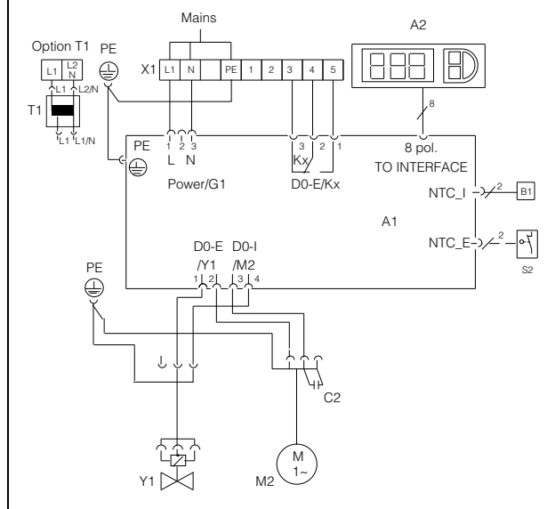
Fig. 17: Schema degli allacciamenti elettrici nr. 1
