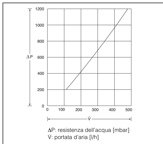
Fig. 37: Resistenza dell'acqua SK 3374.XXX
