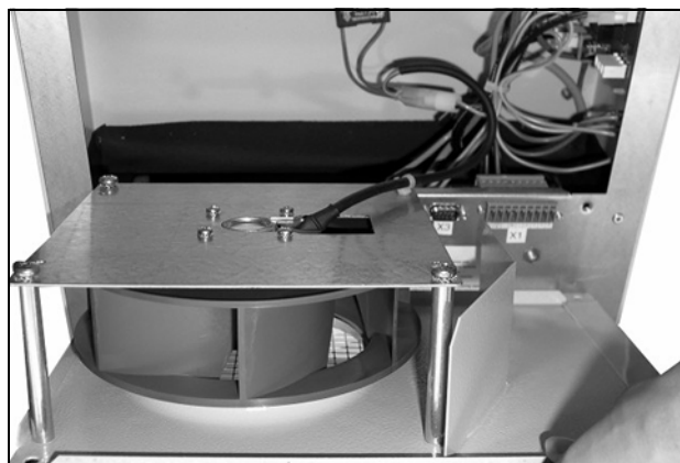
Fig. 29: Togliere la copertura con il ventilatore
