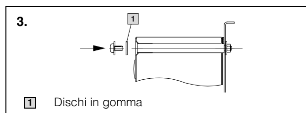
Fig. 7: Fissaggio dell'apparecchio
