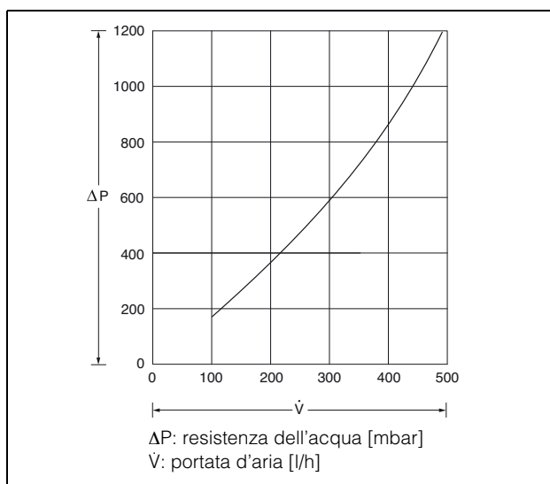
Fig. 36: Resistenza dell'acqua SK 3373.XXX
