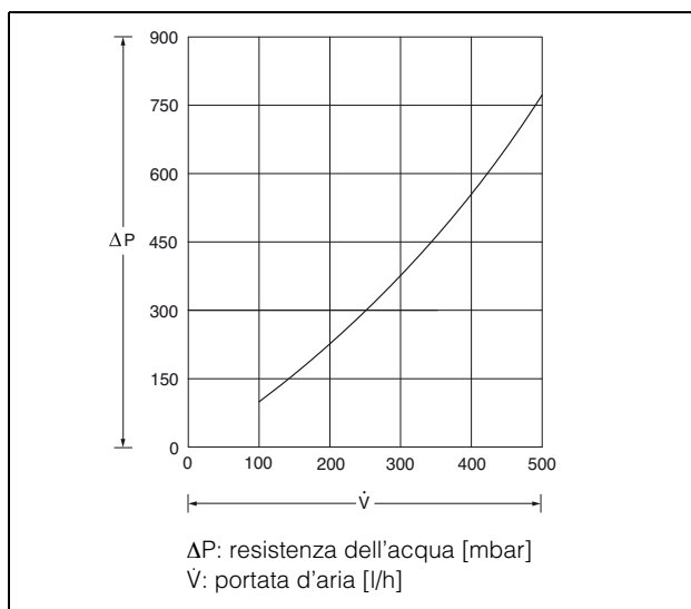
Fig. 34: Resistenza dell'acqua SK 3363.XXX
