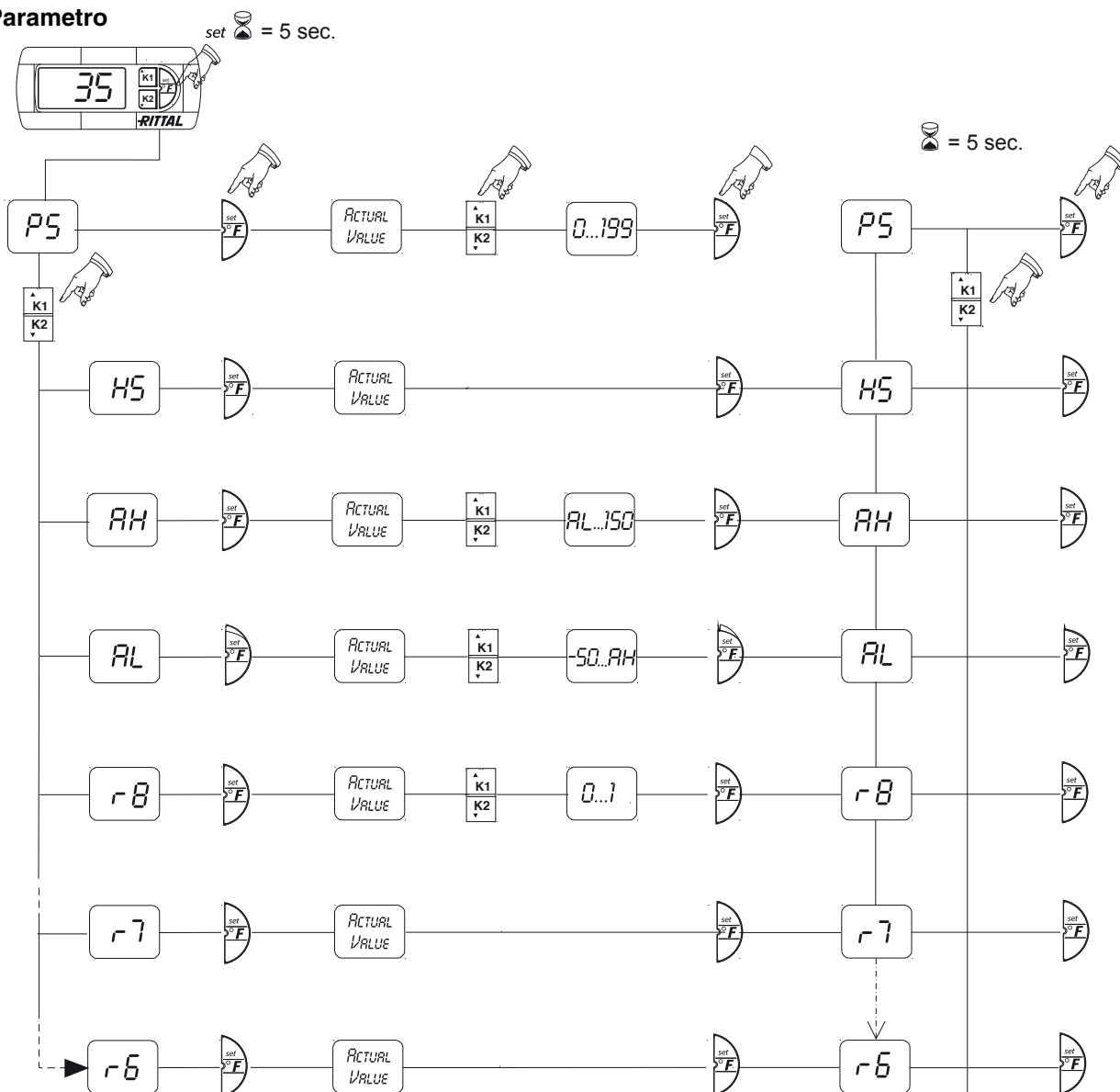
Fig. 20: Schema delle programmazioni del controllo Basic
