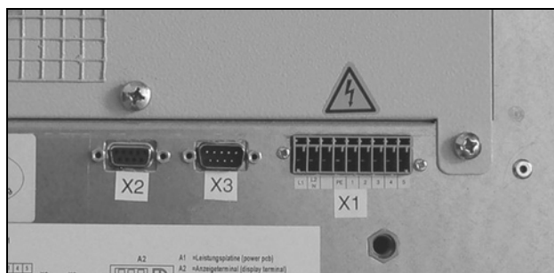
Fig. 27: Estrarre il connettore di alimentazione (X1)
