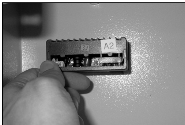
Fig. 30: Estrarre il connettore del display
