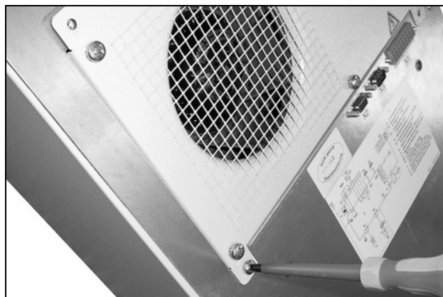
Fig. 28: Togliere le viti di fissaggio della copertura
