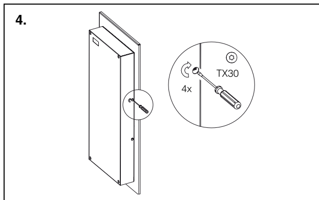
Fig. 8: Avvitare a fondo le viti in senso orario
