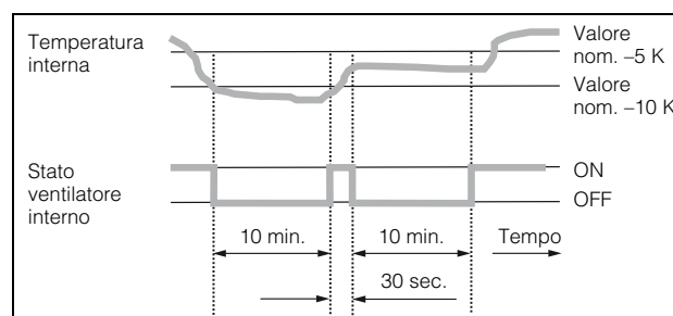
Fig. 22: Grafico Controllo a risparmio energetico Eco Mode
