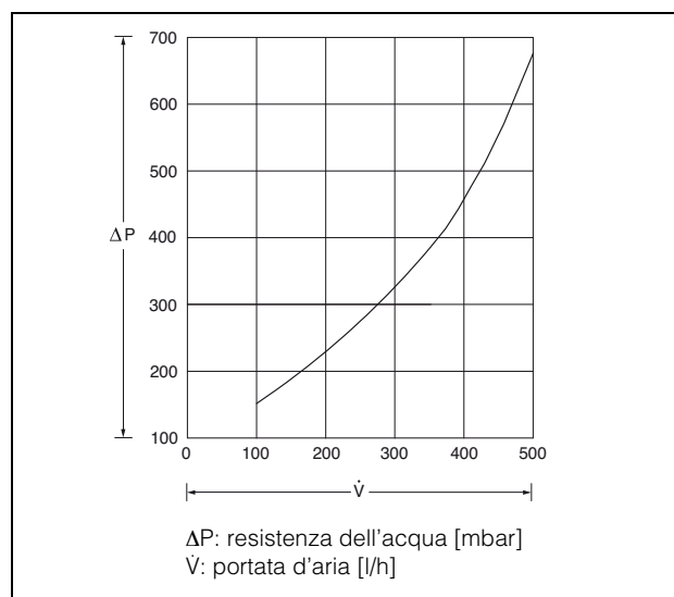
Fig. 38: Resistenza dell'acqua SK 3375.XXX
