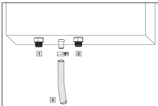
Fig. 14: Collegamento dello scarico di condensa
