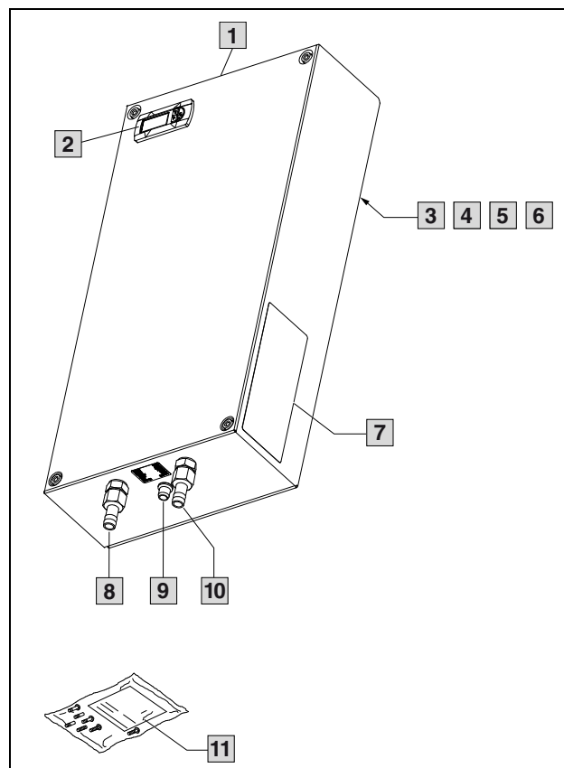
Fig. 1: Descrizione dell'apparecchio
