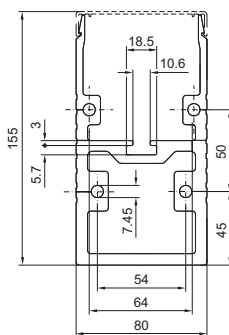
Kannatinprofiili avoin
