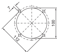
Asennusaukotus, kotelo CP-XL
