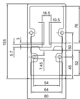
Kannatinprofiili umpinainen
