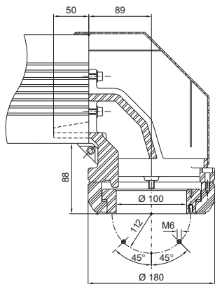
Asennusaukotus, kotelo CP-XL
