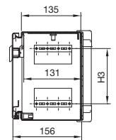
Schnitt A – A
