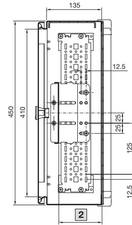
Schnitt A – A
