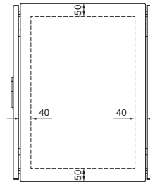
Sección de montaje
