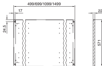
Placa de montaje
