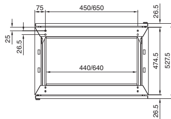
Placa de montaje
