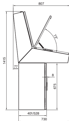
Montaje de 3 piezas
