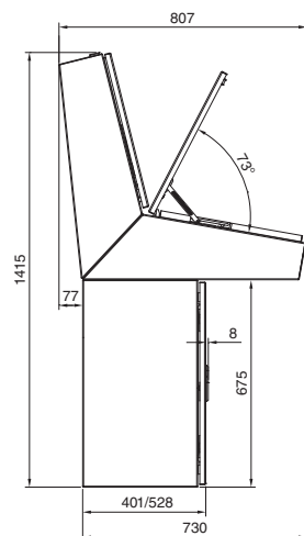
Zabudowa 3-częściowa
