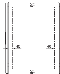
Wykroj montażowy
