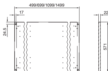
Płyta montażowa
