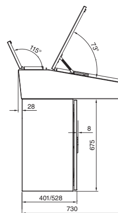
Zabudowa 2-częściowa
