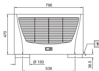
1 Odpyływ kondensatu 1/2", elastyczny
