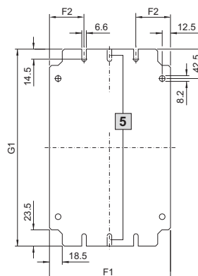
5 Vid 125 mm breda montage- plåtar endast fastsättning i mitten
